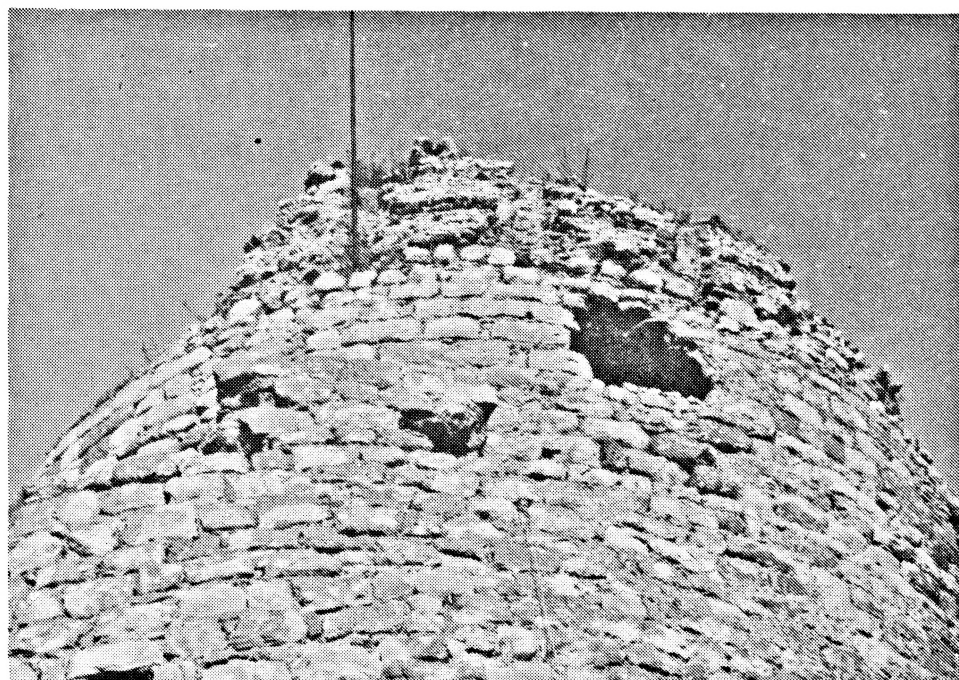
Obr. 5. Michalovice hrad, okr. Mladá Boleslav. Otisk trámové konstrukce na líci posledního patra bergfr.tu. Foto autor.
