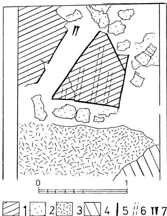
Obr. 8. Týřov hrad, k. ú. Karlova Ves, okr. Rakovník. Část sondy LXII s destruovanou stěnou hrázděného domu. 1 — vypálené bloky mazanicové výplně, 2 — mazanice, 3 — povrch skály, 4 — povrch vrstvy 16, 5 — hrany mazanicových bloků výplně tvořené otiskem dřevěné konstrukce, 6 — dutiny po dřevěných čtyřhranech, 7 — hřeby. Kresba autor.
