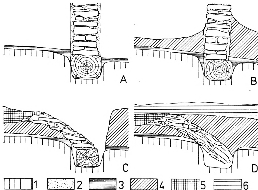
Obr. 6. Angerbach hrad, k. ú. Kožalany, okr. Plzeň-sever. Nádvorní stěna paláce, rekonstrukce postupu destrukce (pominuty epizodické splachy a vrstvičky). A — v průběhu života paláce, B — v procesu pustnutí, C — po vyvrácení zbytku stěny, D — nálezová situace (po vyhníti základového trámu a částečném zvětrání kamenů). 1 — podloží stavby, 2 — jílové pojivo a omítka, 3 — vrstvy životních nečistot, 4 — vyplavené jílové pojivo a omítka s kameny a střešní břidlicí, 5 — hrubá kamenná destrukce, 6 — humózní vrstva a drn. Kresba autor.
