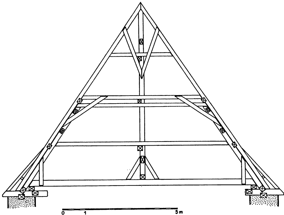
Obr. 18. Brantice, okr. Bruntál. Kostel Nanebevzetí Panny Marie. Schéma plně vazby krovu nad lodí, 1593 a mladší úpravy (D. Prix–M. Zezula, 1999).
