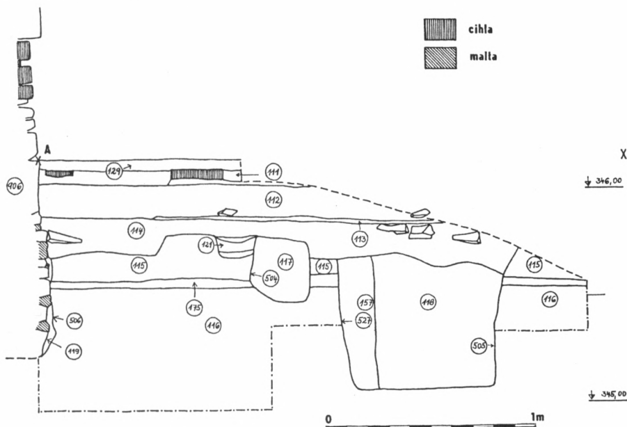
Obr. 10. Brantice, okr. Bruntál. Kostel Nanebevzetí Panny Marie. Profil A–A' v jižní části lodi kostela. Popis: 111 – dlažba z cihel, 112 – dorovnávká terénu, 113 – propálená vrstva, 114 – prachová jílovitá hlína, 115 – tmavý jíl s mazanicí a uhlíky, 116 – podložní jíl, 117 – výplň kůlové jámy 504, 118 – zásyp hrobové jámy 505, 119 – výplň základového vkopu, 121 – spálené dřevo, 129 – maltové lůžko břidlicové dlažby, 157 – zásyp hrobové jámy 527, 175 – zkulturnějším povrchem podloží, 504 – kůlová jáma, 505 – porušená hrobová jáma, 596 – základový vkop pro zeď 906, 527 – hrobová jáma, 906 – jižní zeď lodi kostela.
