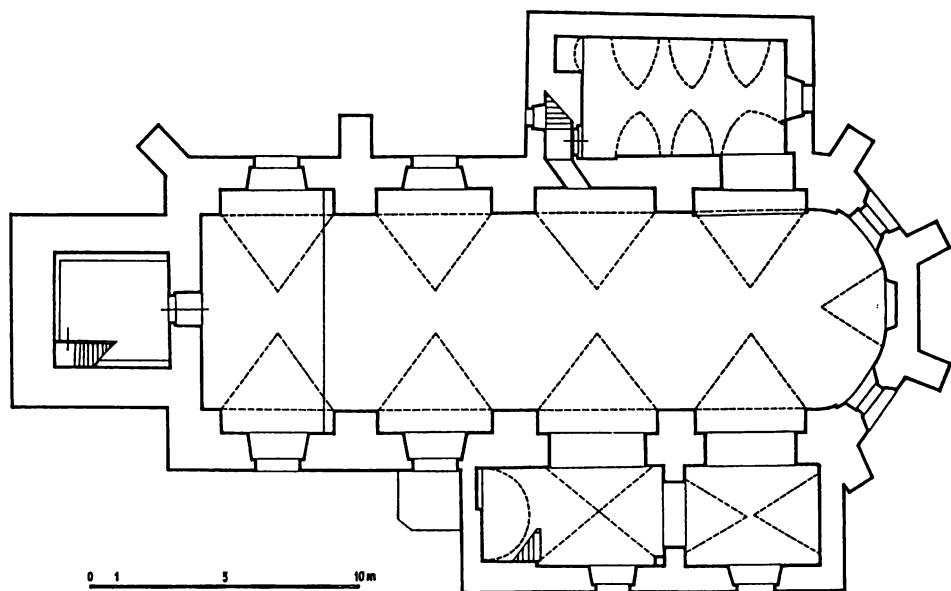
Obr. 23. Brantice, okr. Bruntál. Kostel Nanebevzetí Panny Marie. Půdorys stávajícího stavu v úrovni 1. patra věže. Přerušované vkesleny klenby (D. Prix, 1999).
