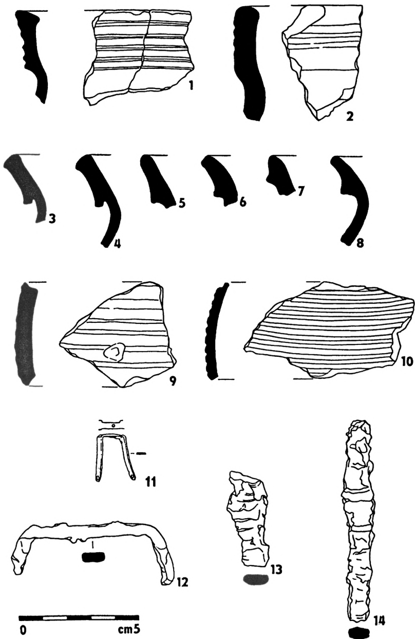
Obr. 11. Brantice, okr. Bruntál. Kostel Nanebevzetí Panny Marie. Výběr nálezů z hrobových zásypů (1–3, 7, 11–14) a starší část stratigrafie chrámového interiéru (4, 8–10: keramické střepy z propálené vrstvy). Kreslila Il. Pravdová.
