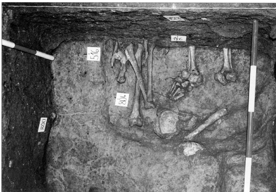
Obr. 14. Brantice, okr. Bruntál. Kostel Nanebevzetí Panny Marie. Jižní kaple: částečně odkrytý pohřeb 804 v původním exteriéru kostela s pietně uloženými kostmi z porušeného staršího pohřbu (M. Zezula 1999).
