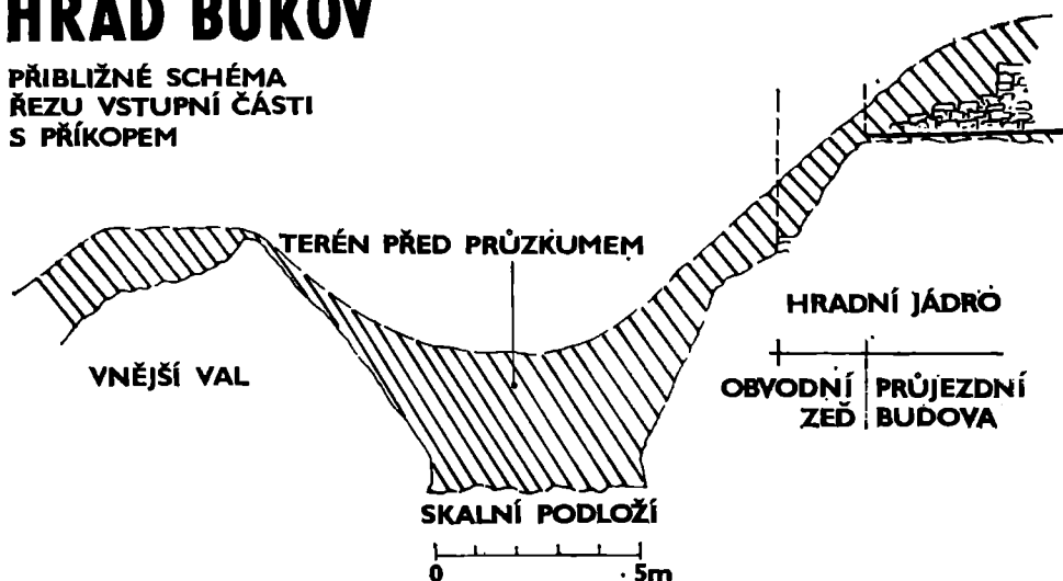
II. Hrad Bukov, přibližné schéma řezu vstupní části s příkopem . Podle L. J. Konečného nakreslila I. Kucharská
