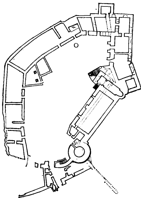
V. Hrad Znojmo, půdorys vnitřního hradu . Podle zaměření z 2. desetiletí 18. století (srov. obr. příl. 45) nakreslila I. Kucharská
