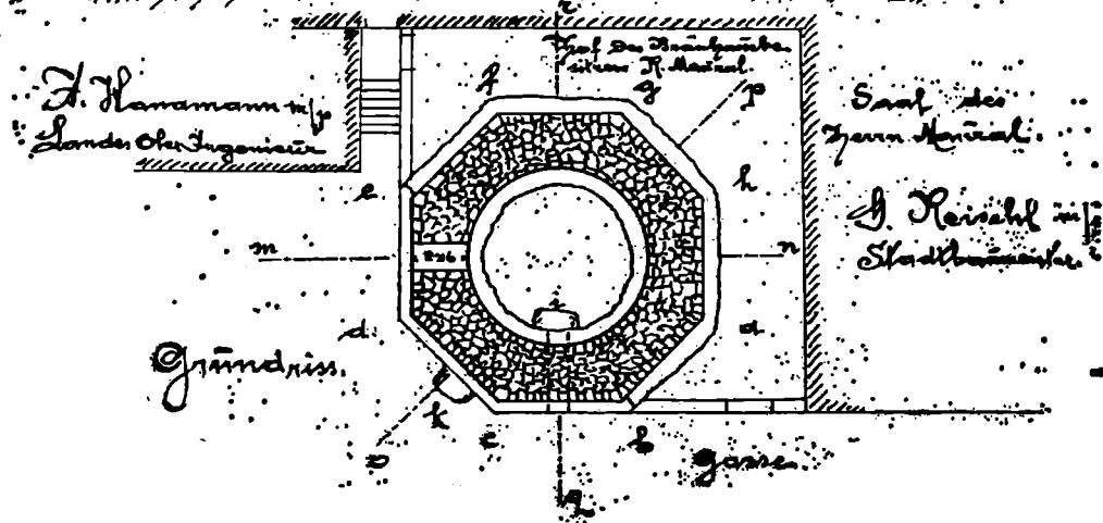
VI Znojmo, hrad, tzv. Loupežnická věž, půdorys a řezy. Zaměřili a nakreslili A. Hanamann a H. Reischl (1889)
