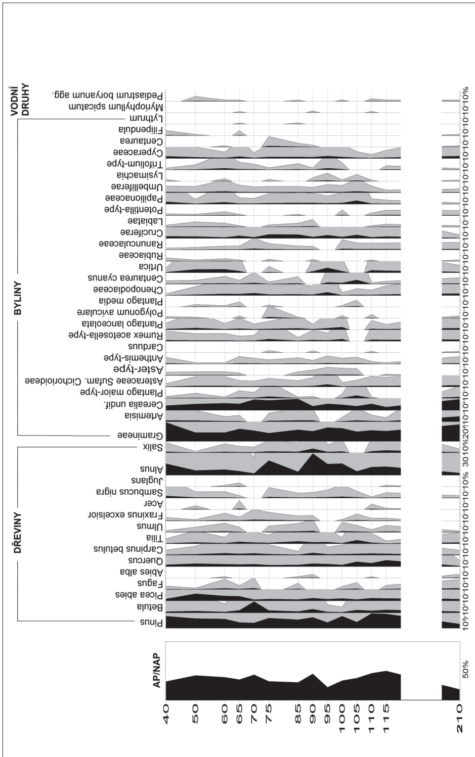
Obr. 5. Palynogram k vrtu Jevišovka.
