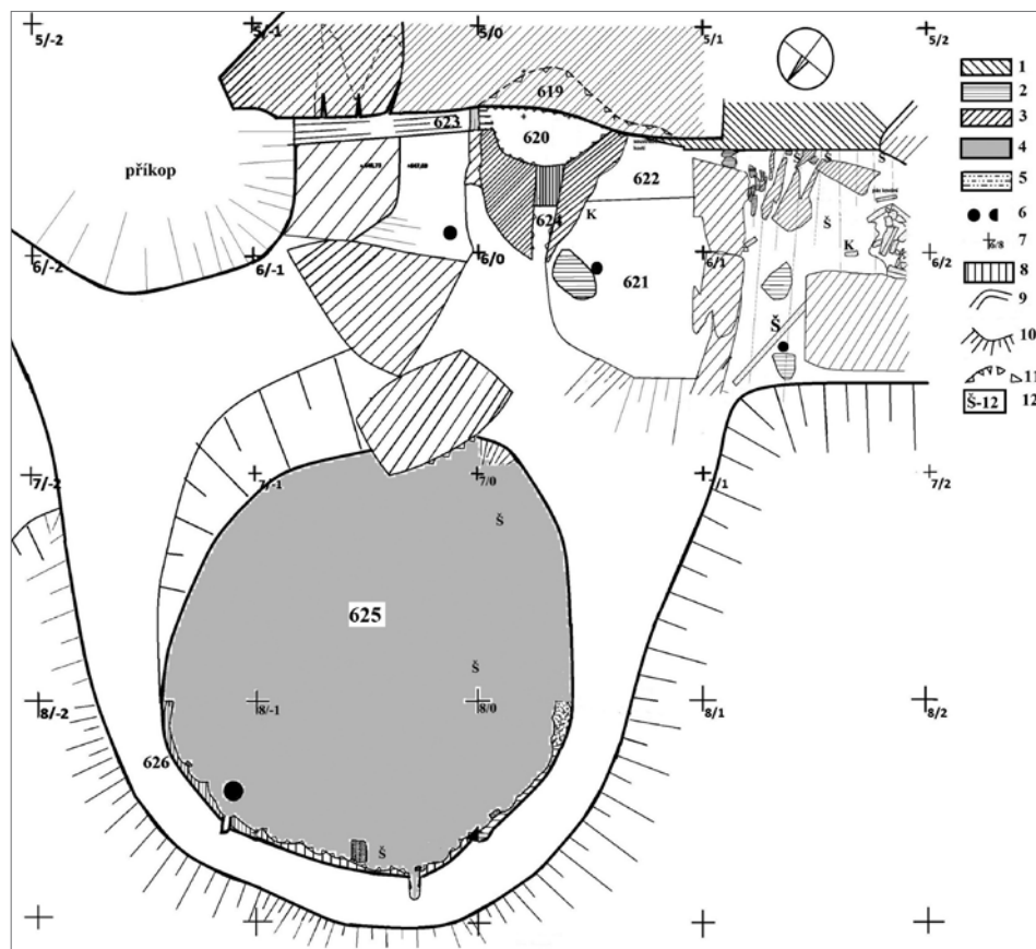
Obr. 11. Půdorysné zobrazení severního nároží hradu s vyznačením objektů a některých nálezů. 1 – zdívno, 2 – kameny, 3 – skála a oddělené kusy skal, 4 – kruhové obranné postavení, 5 – dřevo, 6 – dělové koule a jejich části, 7 – body čtvercové pětimetrové sítě, 8 – jíl, 9 – vrstevnice, 10 – sklon terénu, 11 – hrany terénu a vyznačení zahloubení otvoru ve skále. Nálezy: Š – šípky, K – olověné projektily. Objekty: 619 – otvor do skály, 620 – nádržka, 621, 622 – srovnaná plocha, 623 – přítokový kanál, 624 – odtokový kanál, 625 – kruhové opevnění.
