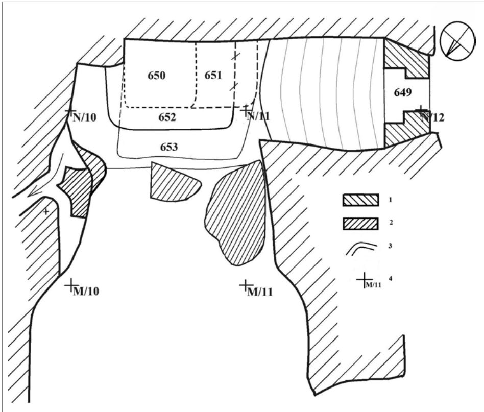
Obr. 14. Půdorysné zobrazení plochy vápenky s vyznačením objektů (obr. 1:9). 1 – zdivo, 2 – skála a oddělené kusy skal, 3 – vrstevnice, 4 – body čtvercové pětmetrové sítě. Objekty: 649 – vstup, 650 – vrstva čistého vápna, 651 – vrstva znečištěného vápna, 652 – zpevněná podlaha, 653 – podklad podlahy.
