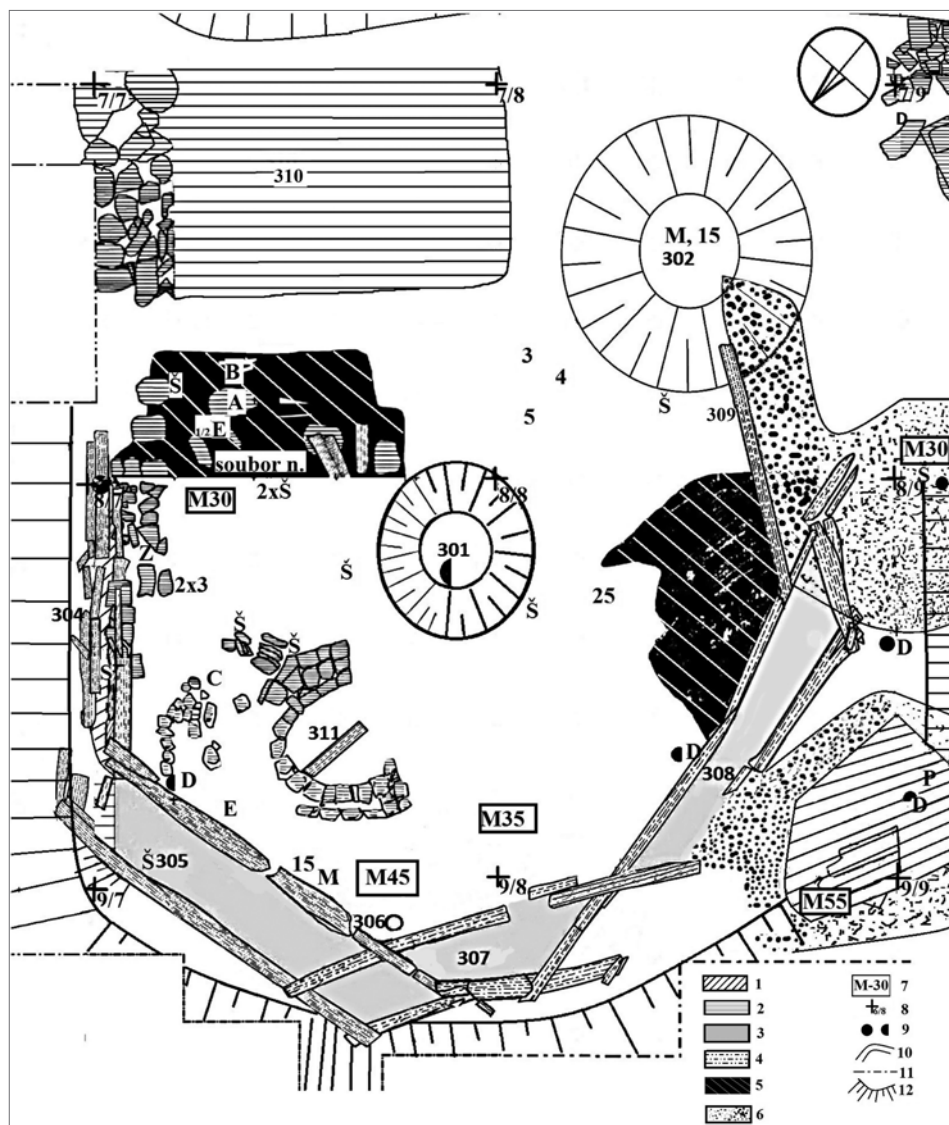
Obr. 3. Půdorysné zobrazení dřevohlinité bašty s vyznačením objektů a některých nálezů. 1 – skála, 2 – dlažba a jednotlivé kameny, 3 – hlinitopískitá výplň stěn bašty, 4 – dřevěná výplň, 5 – spáleniště, 6 – mazanice, hustota bodů dle jejího množství, 7 – vyznačení mocnosti mazanice v centimetrech, 8 – body čtvercové pětmetrové sítě, 9 – dělové koule a jejich části, 10 – vrstevnice, 11 – výkopové hrany, 12 – sklon terénu. Nálezy: A – hrnec, B – pohár, C – kahánek, D – dělové koule a jejich části, E – poklice, M – mince, P – podkova, Š – šipka s tulejí, Z – visací zámek, 3 – nůž, 4 – sekáč, 5 – knoflík, 15 – kroužková zbroj, 25 – velký hřeb. Soubor zahrnuje kování dveří, závorovou skobu, západku zámku, dva závěsy dveří a postranici. Objekty: 301, 302 – kruhové jámy, 304, 305, 307, 308 – stěny bašty, 306 – kulová jamka.
