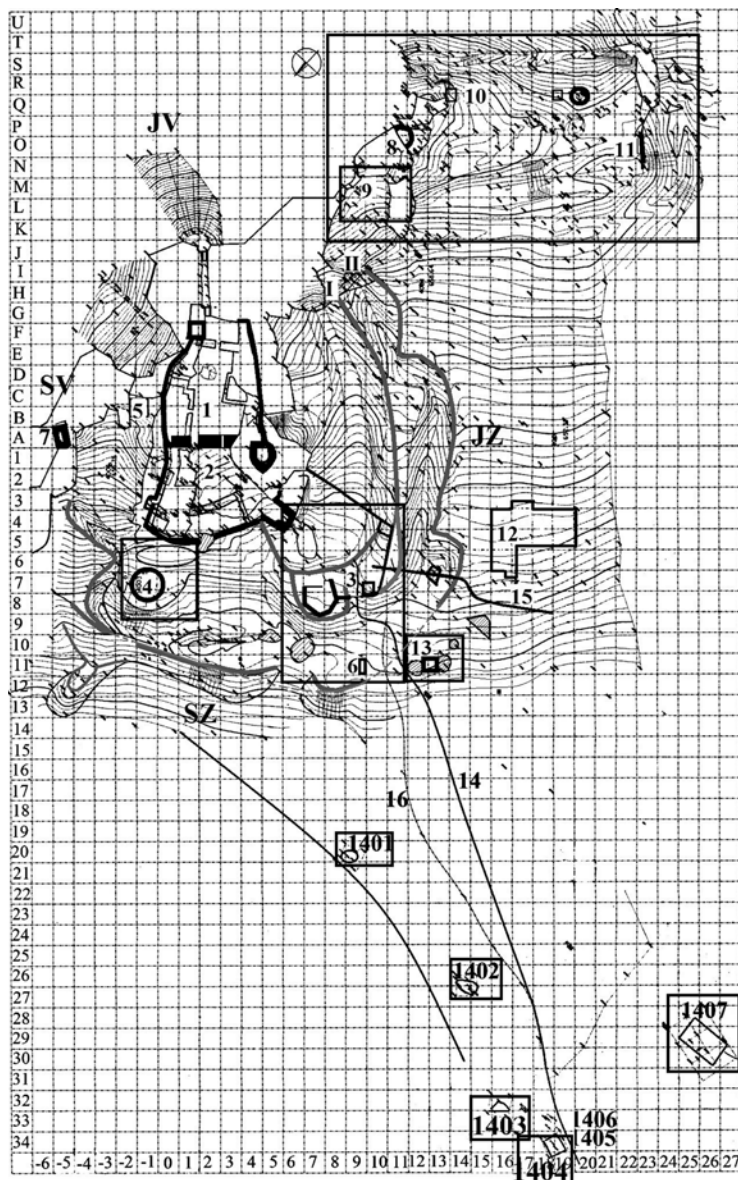
Obr. 1. Půdorysné zobrazení hradu Skály a objektů před ním. 1 – jádro hradu, 2 – druhé předhradí, 3 – první předhradí, 4 – opevnění severního nároží, 5 – dílna na měděné výrobky, 6 – kovárna na barevné kovy, 7 – severovýchodní předsunutá věž, 8 – jižní předsunutá věž, 9 – vápenka, 10 – opevněné návrší, 11 – dřevohlinitá stěna, 12 – kovárský areál, 13 – předsunutý srub, 14 – přístupová cesta do hradu, 15 – původní přístupová cesta do hradu, 16 – dnešní cesta, 1401, 1402, 1404–1406 – předsunuté zahloubené sruby, 1403, 1407 – obléhací postavení, I, II – valy. Šedě zvýrazněny průběhy valů: tenká čárková linie – zrušené úseky, silná linie – současný stav. Po obvodu vyznačení číslování čtverců v síti 5 × 5 m a ve vyobrazení body výškového zaměření. Kresba Ing. D. Šiler.
