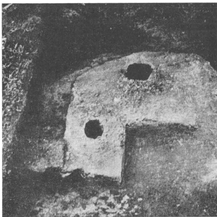
Obr. 2. Pohled na zahlobené nistěje peci, Olomučany, okr. Blansko.
