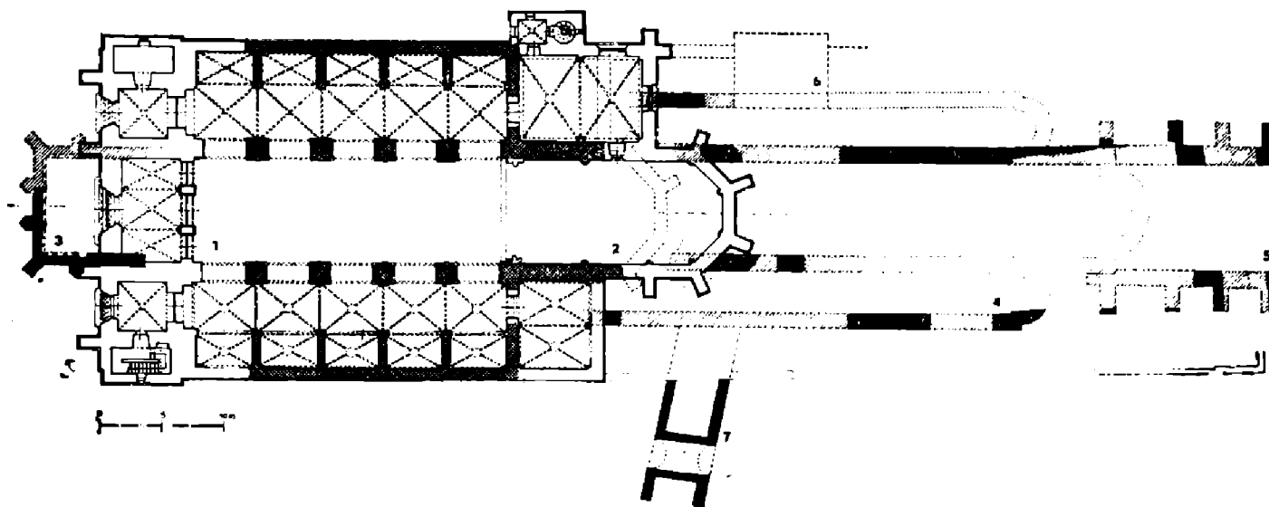
Obr. 1. Půdorys kostela sv. Petra a Pavla na Vyšehradě v rekonstrukci středověkého stavu na základě výsledků archeologického výzkumu: — řídké mřížky značí středověké zdivo nad terénem (včetně části rekonstruovaných J. Mockerem) — husté mřížky — zaniklé středověké zdivo známé nebo zjištěné výkopem (včetně zdiva zjištěného v negativu), šikmá šrafura — dotvořený průběh zdiva mezi sondami. — 1 půdorys dnešního kostela, 2 — pozdně gotický případně renesanční kostelní závěr, zbořený při regotisaci, 3 — zaniklá gotická síň před západním průčelím kostela, 4 — nalezená apsida románské jižní lodi, 5 — závěr chrámu ze 14. století, 6 — situace bývalé zvonice.
