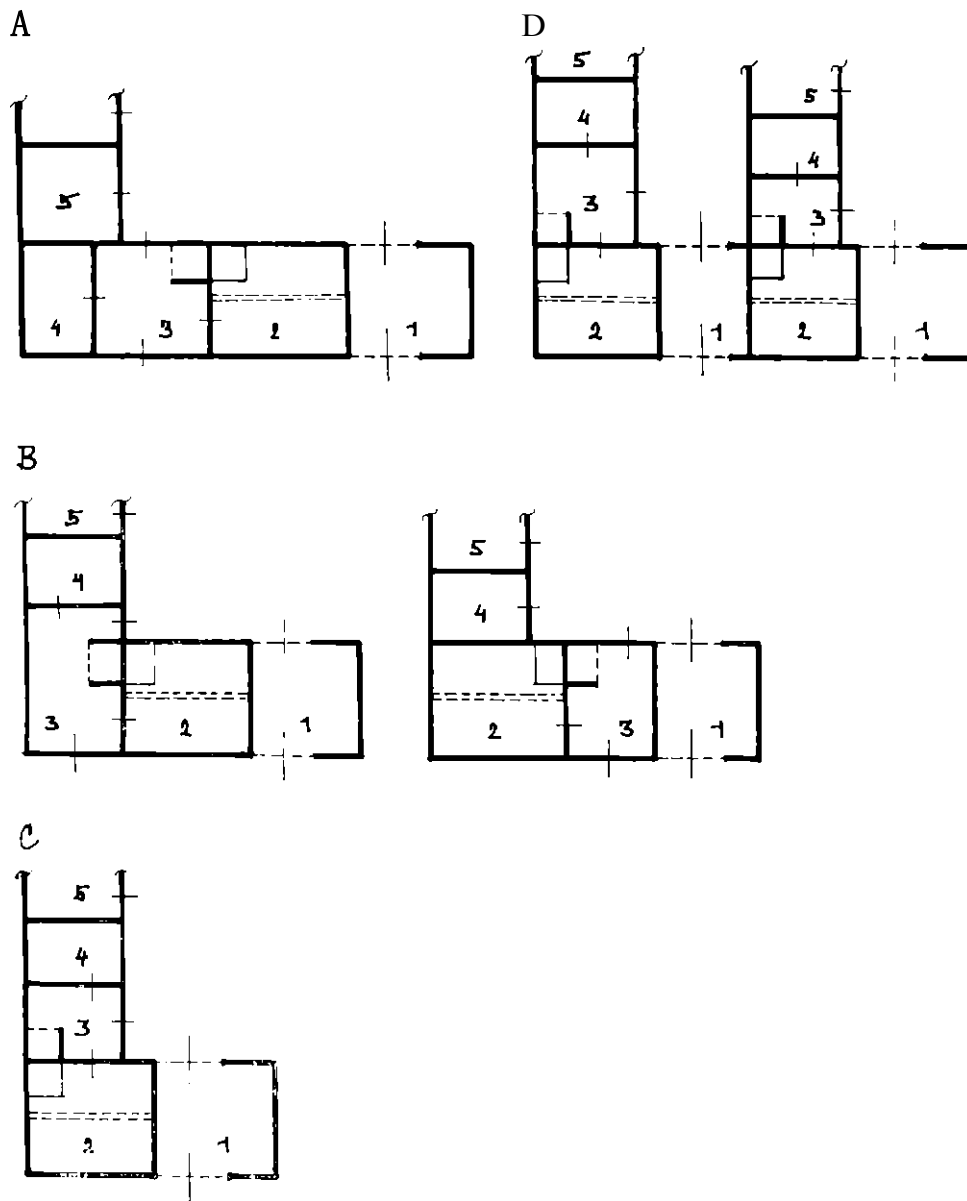
Obr. 2. Strážnice. Ideální schéma základních typů lidových objektů. 1 – průjezd (navráti či miatevna), 2 – světnice, 3 – sín s černou kuchyní, 4 – komora, 5 – chlév. – A) Nejrozšířenější typ dispozice na parcelách s největší šířkou. B) „Přechodný“ typ na užších parcelách. C) Typ převažující na nejdíších parcelách. D) Informativní příklad dělení objektu, které je typické zejména pro 19. století (viz úvodrys A).
