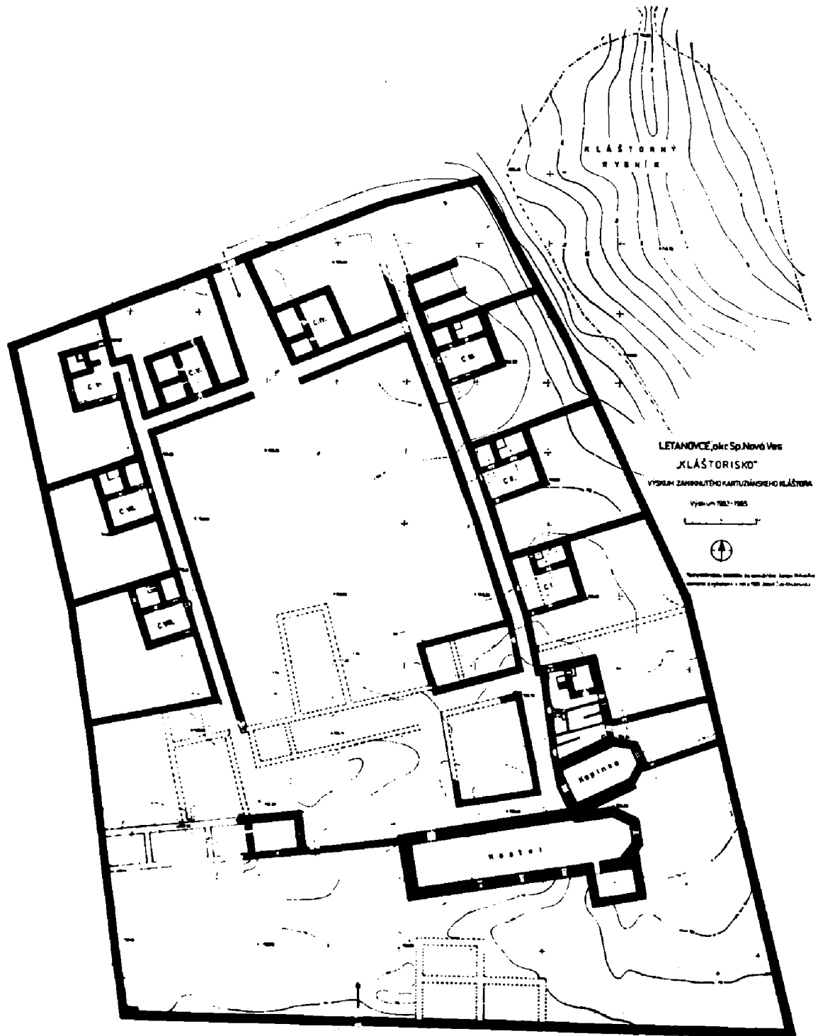
Obr. 3. Predbežný pôdorys kartuziánskeho kláštora.
