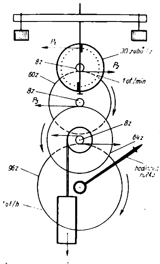
Obr. 6. Schéma přenosu sil v luhýfových hodinách. Podle St. Michala.
