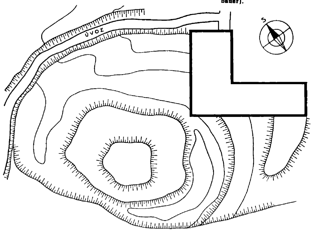
Obr. 13. Oldřichov — půdorys (tvrz (zaměřil Zd. Rothbauer).
