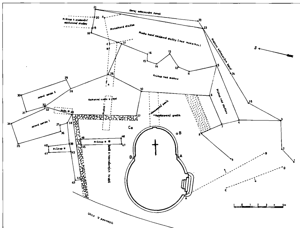
Obr. 4. Rotunda sv. Martina na Vyšehradě – plán archeologického výzkumu K. Gutha z let 1924–1926.
