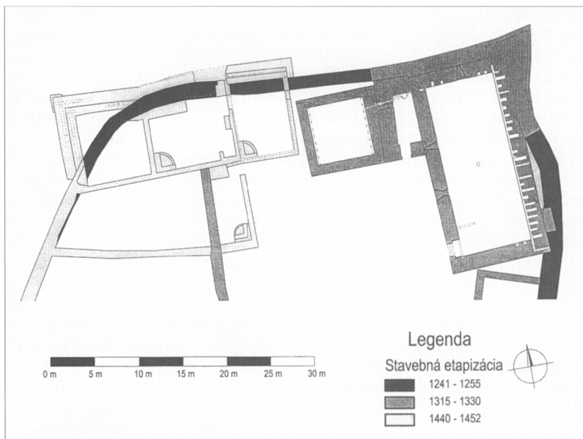
Obr. 4. Zvolen – Starý Zvolen (Pustý hrad). Stavebná etapizácia Dončovej časti hradu z rokov 1241–1452. Zamerali: M. Bábik, Ing. arch. P. Surovec.
