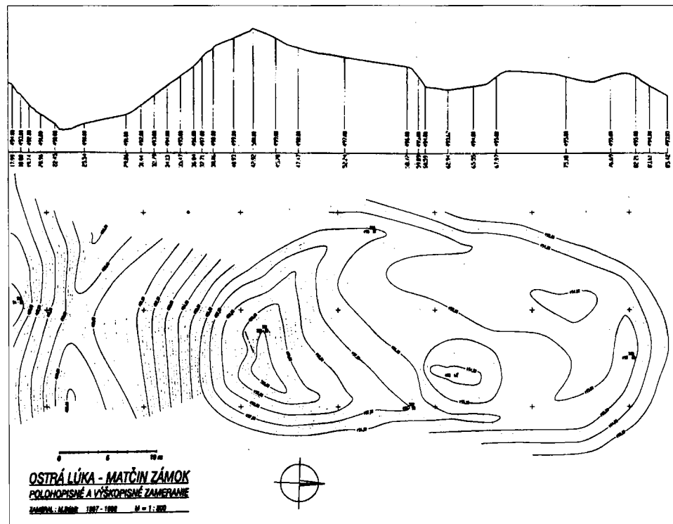
Obr. 8. Ostrá Lúka - Matčín zámok. Výškopisné zameranie opevnenej polohy datovanej k roku 1451. Zamerateľ: M. Bábik.
