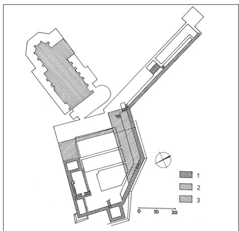
Obr. 3. Hrádek na Zderaze na Novém Městě pražském. Nahoře vlevo hrad na veduté z Liber chronicarum Hartmanna Schedela z roku 1493, vpravo na veduté J. Sadelera z roku 1606. Dole vlevo půdorysná rekonstrukce hradu zakreslená do obrysu zástavby na počátku 20. století. 1 – zdivo hradu dochované počátkem 20. století, 2 – rekonstruované součásti hradu, 3 – gotický rozsah kostela Sv. Václava na Zderaze (kresba autor). Vpravo přestavěný hrad se Svatováclavskou trestnicí na fotografii z roku 1884.
