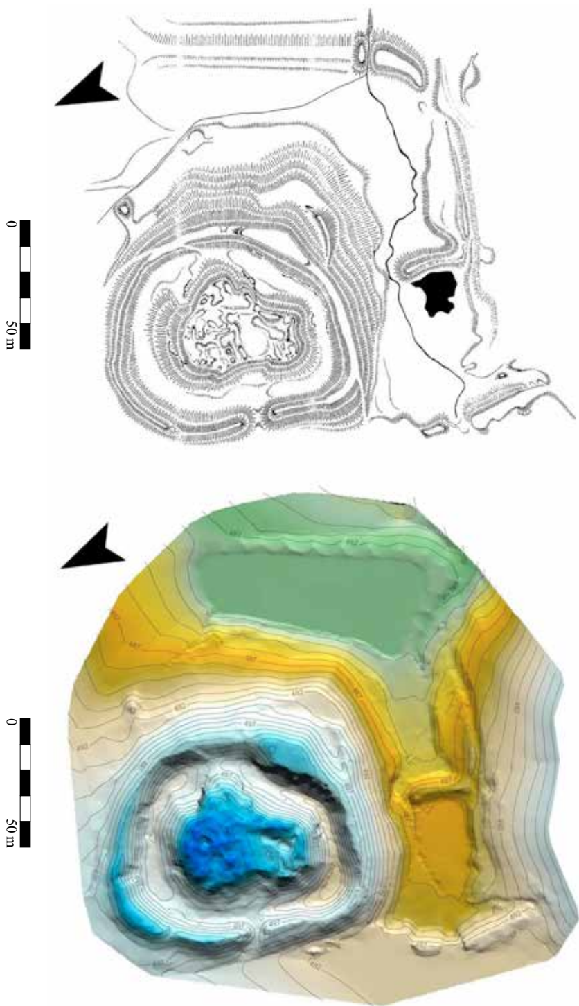
Obr. 4. Srovnání plánů lokality: Vlevo plán J. Anderleho a J. Milera z roku 1982, vpravo plán na základě měření z let 2010–2011. Abb. 4. Vergleich der Fundstellenpläne: Links Plan von J. Anderlý und J. Miler aus dem Jahr 1982, rechts Plan auf Grundlage der Vermessung aus den Jahren 2010–2011.
