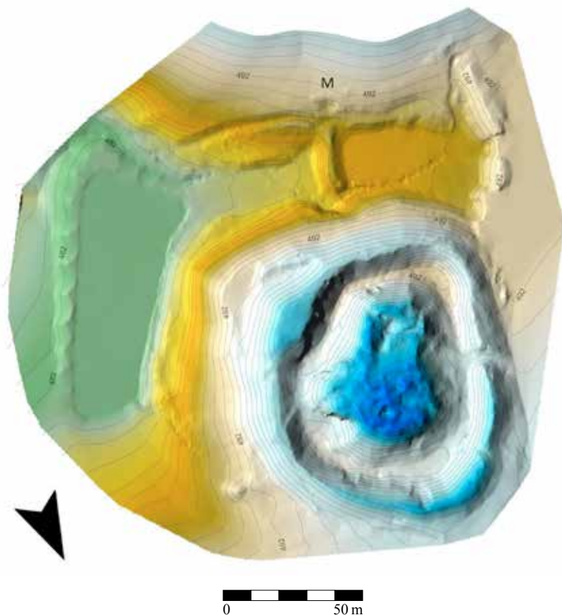
Obr. 3. Plán lokality 3D s vyznačením vrstevnic. M – pozice relikvů mlýna. Abb. 3. 3D-Plan der Fundstelle mit Höhenschichtlinien. M – Lage der Mühlenrelikte.
