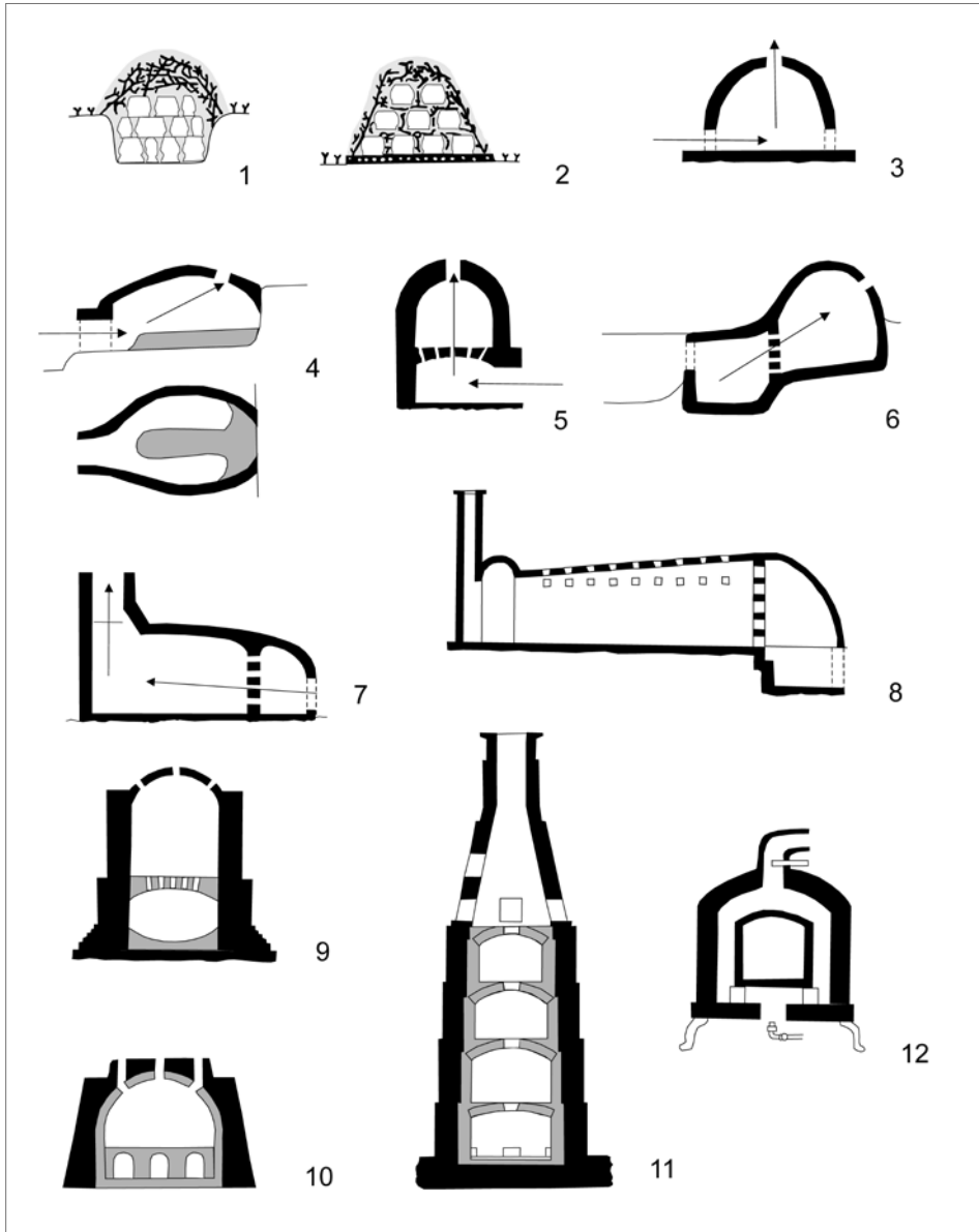
Obr. 13. Přehled typů vypalovacích zařízení a hrnčářských pecí. 1 – otevřený výpal na způsob milře (podle Henderson 2000, Fig. 4.11, 1); 2 – jámový otevřený výpal (podle Henderson 2000, Fig. 4.11, 2); 3 – jednoprostorová vertikální pec (podle Volf 2006, příl. 17:1); 4 – ležatá pec se středovým jazykem (podle Volf 2006, příl. 17:IV); 5 – vertikální (stojatá) pec (podle Kaltenberger 2009, Abb. 402); 6 – horizontální dvouprostorová pec s dělicí přepážkou (podle Janssen 1987, Abb. 17); 7 – horizontální (ležatá) pec (podle Kaltenberger 2009, Abb. 409); 8 – kasselská pec (podle Heege 2007, 40); 9 – obdélníkovitá pec na majoliku/fajáns (podle Heege 2007, Abb. 89); 10 – pec na kameninu (podle Kaltenberger 2009, Abb. 416); 11 – poschodová pec na porcelán (König et al. 2011, Abb. 8); 12 – muflová plynová pec (podle Rada 1956, obr. 215). Sestavil L. Čapek.
