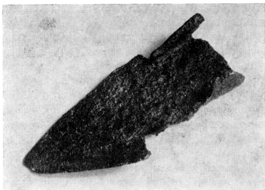
Obr. 10 Tisová (okr. Jistebnice). Asymetrická radlice z nálezů ve dvoře. Foto: Fr. Cáp.
