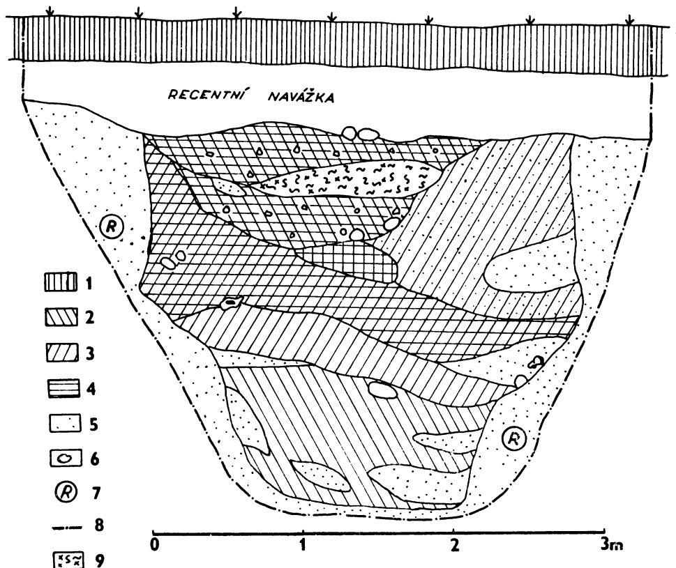
Obr. 1. Přibice. Rez středověkou jámou. 1 – ornice, 2 – černá hlína, 3 – šedá hlína, 4 – hnědá hlína, 5 – písek, 6 – kameny, 7 – rostlý terén, 8 – hranice řezu, 9 – struska a uhlíky.
