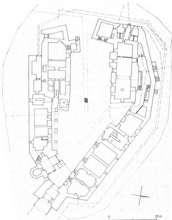
Obr. 2. Blatná hrad, okr. Strakonice. Půdorys současného stavu přizemí se zakreslenými výkopy inženýrských sítí z roku 1976. Čerchované provedené rýhy, které nebylo možno dokumentovat, tečkované obrýsy dokumentovaných výkopů, černě nově zjištěné záivo. Kresba P. Chotěbor.
