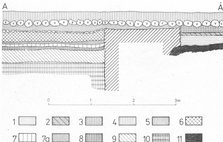
Obr. 6. Blatná hrad, okr. Strakonice. Průkop nádvořím, profil A. Zdivo šrafováno silněji. 1 – rostlý písčité terén, 2 – černé spáleniště, 3 – písčité navážka, 4 – písčité, 5 – žlutavé písčité, 6 – bělavé písčité s maltovinou, 7 – žlutavé písčité, 7a – tmavší žlutavé písčité, 8 – tmavá masná, 9 – písčité s uhlíky, 10 – hnědá písčité, 11 – skála. Kresba J. Durdíková.
