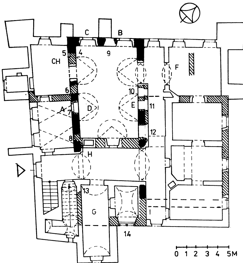
Obr. 3. Bratislava — Devín, kaštieľ na Hutníckej ul. č. 25. Pôdorys prízemlia, stavebno-historická analýza. Čierne murivo I. etapy, šrafované murivo II. a III. etapy, 4. ostenie okna z I. etapy, 5. okno z III. etapy, 6. otvor z II. etapy, 7. portál z III. etapy, 8. vetrací otvor z I. etapy, 9 až 12, otvory z III. etapy, 13. portál z III. etapy, 14. okno s paspartou z III. etapy. Písmenami A—I sú označené archeologické sondy.
