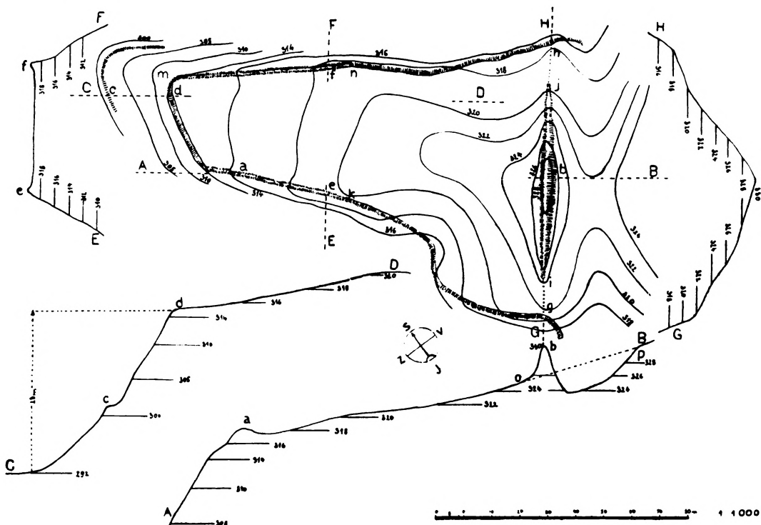
Obr. 1. Zvolen — hradisko Priekopa. Plán lokality s výškopisným zameraním a rezmi od Š. Janáka.
