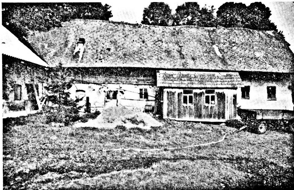
Obr. 3. Čistá čp. 171, dvortkové průčelí domu s novodobou verandou před vstupem a odřezanou pavlačí u zadní patrové části. Vlevo mladší kolmé hospodářské křídlo. Foto J. Škabrada, 1988.
