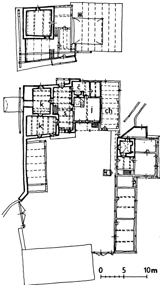
Obr. 8. Čistá čp. 12, půdorys usedlosti podle V. Mencla, dole přízemí, nahoře patro domu. s – vstupní síň, l – lizba, č – černá kuchyně, k – komory, ch – chlév, přistavěný dodatečně před čelní stěnu lizby.
