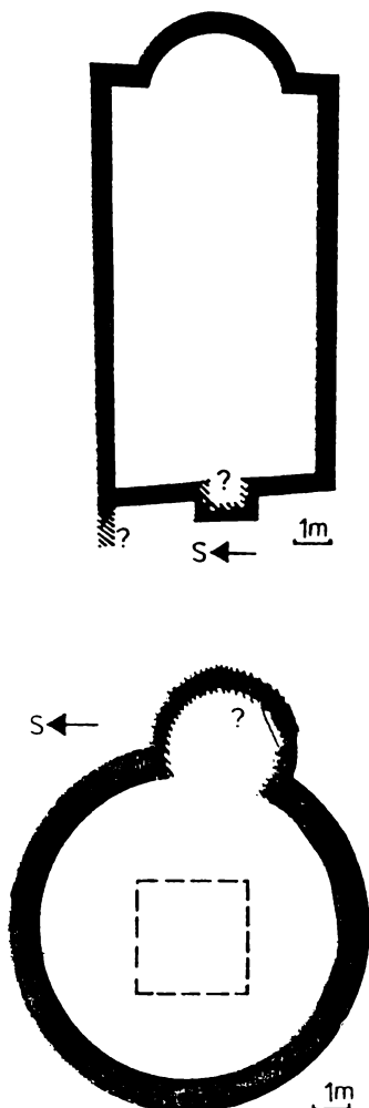
Obr. 5. Praha 2, Vyšehrad — detail zaměření jednoduchého kostelíka a kruhové stavby (podle J. Vydry a P. Starce).
