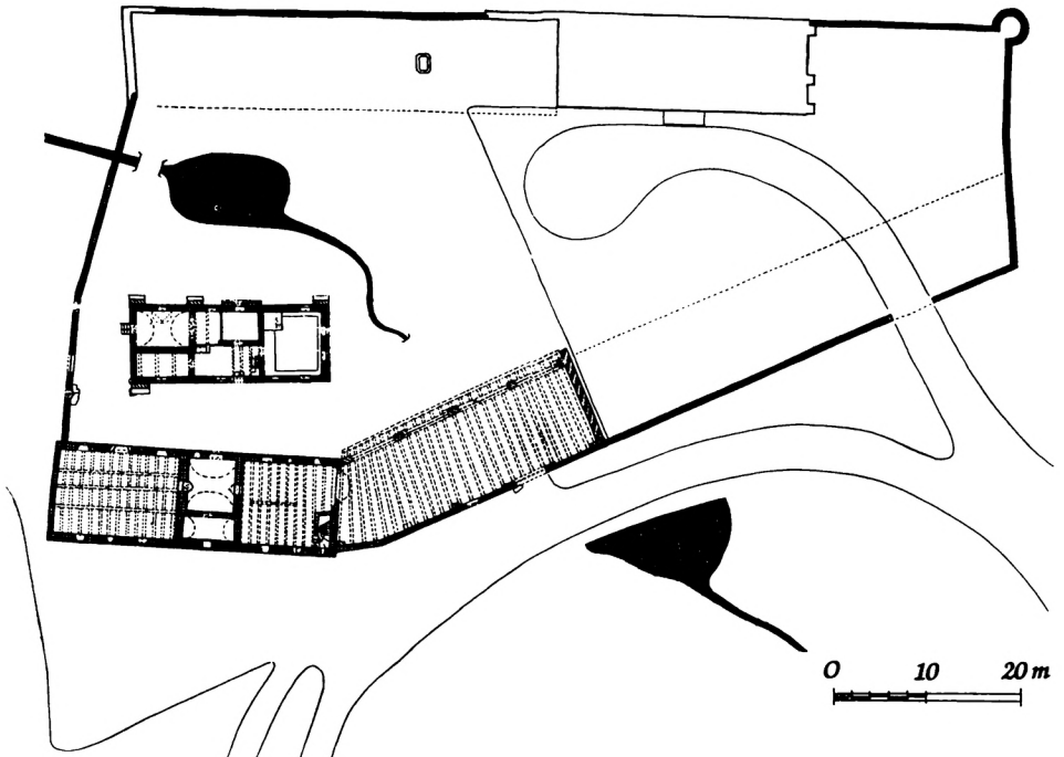
Obr. 9. Holešice, o. Písek, půdorys, zpracovaný podle zaměření v archivu Památkového ústavu v Českých Budějovicích, se stavebně historickou analýzou.
