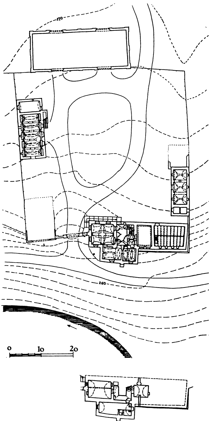
Obr. 2. Hořenice u Jaroměře, o. Náchod, dvorec ép. 1. Skica půdorysu přízemí s odvozenými vrstevnicemi a sklepa podle stavu v roce 1985.
