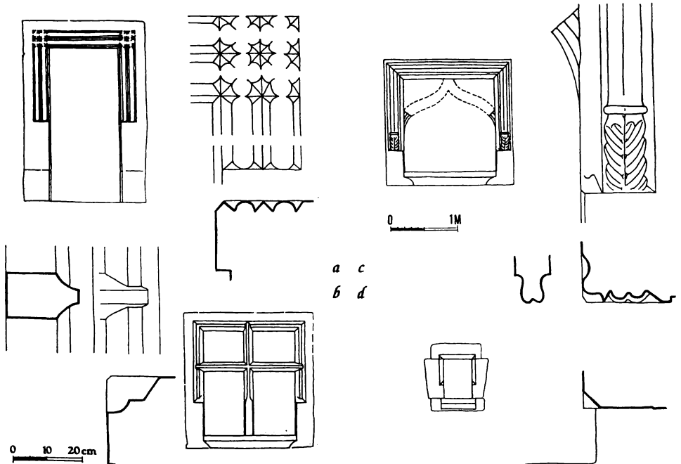
Obr. 4. Zaječice, o. Chrudim, obytné stavení, čp. 1 — portál (a), okno v přízemí (b) a v patře (c), na východním a okénko (d) na jižním průčelí obytného stavení, čp. 1. Měřítko všech celkových nárysů i všech podrobností jsou shodná.
