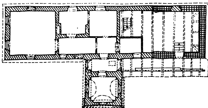
Obr. 5. Míkovice, o. Benešov, 1. a 2. podlaží tvrze podle stavu v roce 1992 se stavebně historickou analýzou; křížkované zdivo renesanční, šrafované barokní a tečkované novodobé. Stejného značení (spolu s klasicistním zdivem dvojitě šrafovaným) je použito i v dalších půdorysech.
