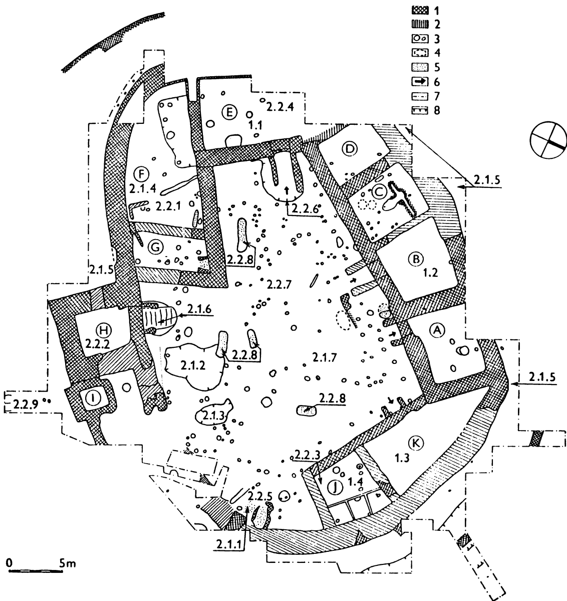
Obr. 1. Plán vnitřního hradu s vyznačením nálezových celků. Legenda: 1 — dochované zdivo, 2 — zdivo v negativu, 3 — kulevé jamky, 4 — nejasná hranice, 5 — propáleno, 6 — vstupy, 7 — hranice zkoumané plochy, 8 — hranice svahu.
