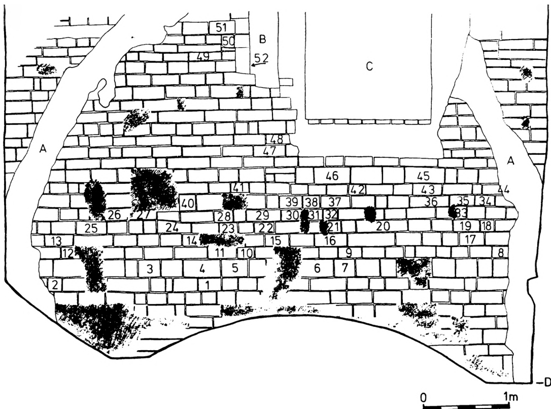
Obr. 1. Rozmístění rytin na jižní stěně věže. 1–52 kvádříčky s rytými kresbami, A — dodatečně zadržaná jizva po odstraněné románské klenbě, B — otvor románské střílny, C — dodatečně upravená nika, D — předpokládaná úroveň podlahy. Stínované dodatečně drobné zásahy do románského zdiva. Zaměření J. Mourek, J. Vejnarová, kresba J. Mourek.
