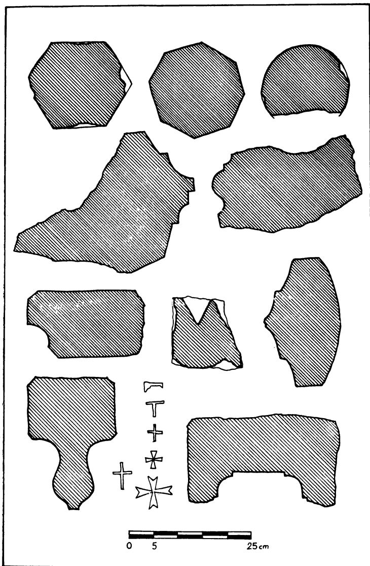
Obr. 4. Pražský hrad, klášter sv. Jiří. Výběr z dokumentace architektonických článků druhotně zazděných ve zdivu barokní kvadratury.
