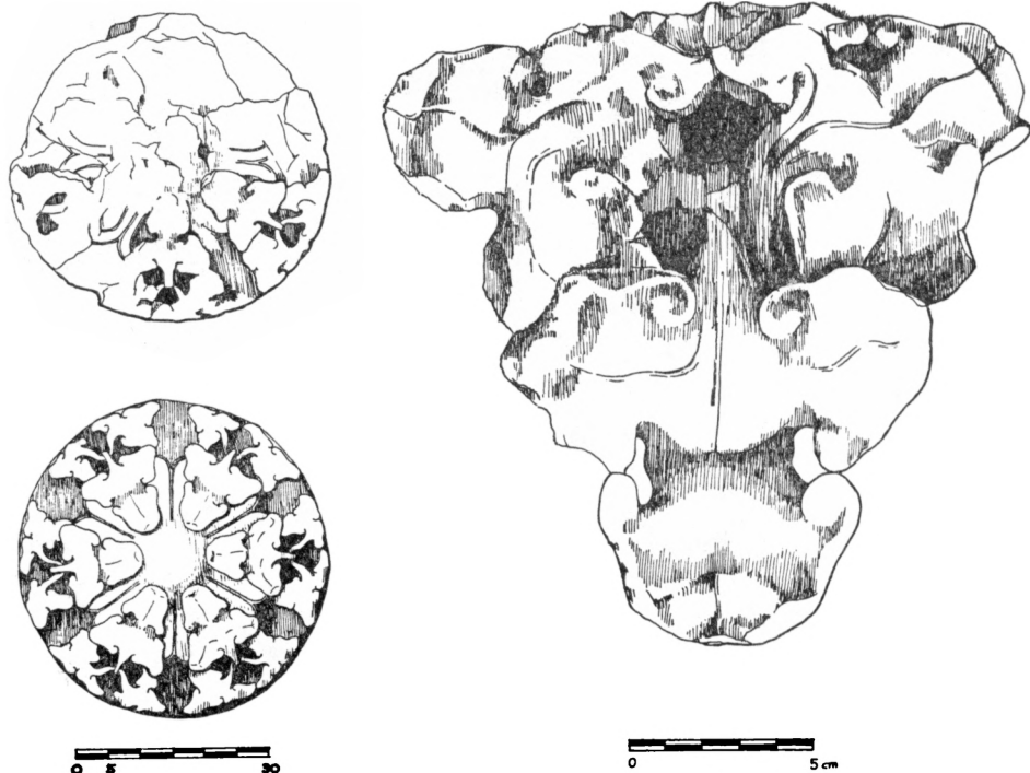
Obr. 7. Pražský hrad, klášter sv. Jiří. Gotický svorník. Nahoře náleзовý stav, dole rekonstrukce. Obr. 8. Pražský hrad, klášter sv. Jiří. Detail trojice trojlaločných listů z výzdoby gotického svorníku. Všechny kresby P. Chotěbor.
