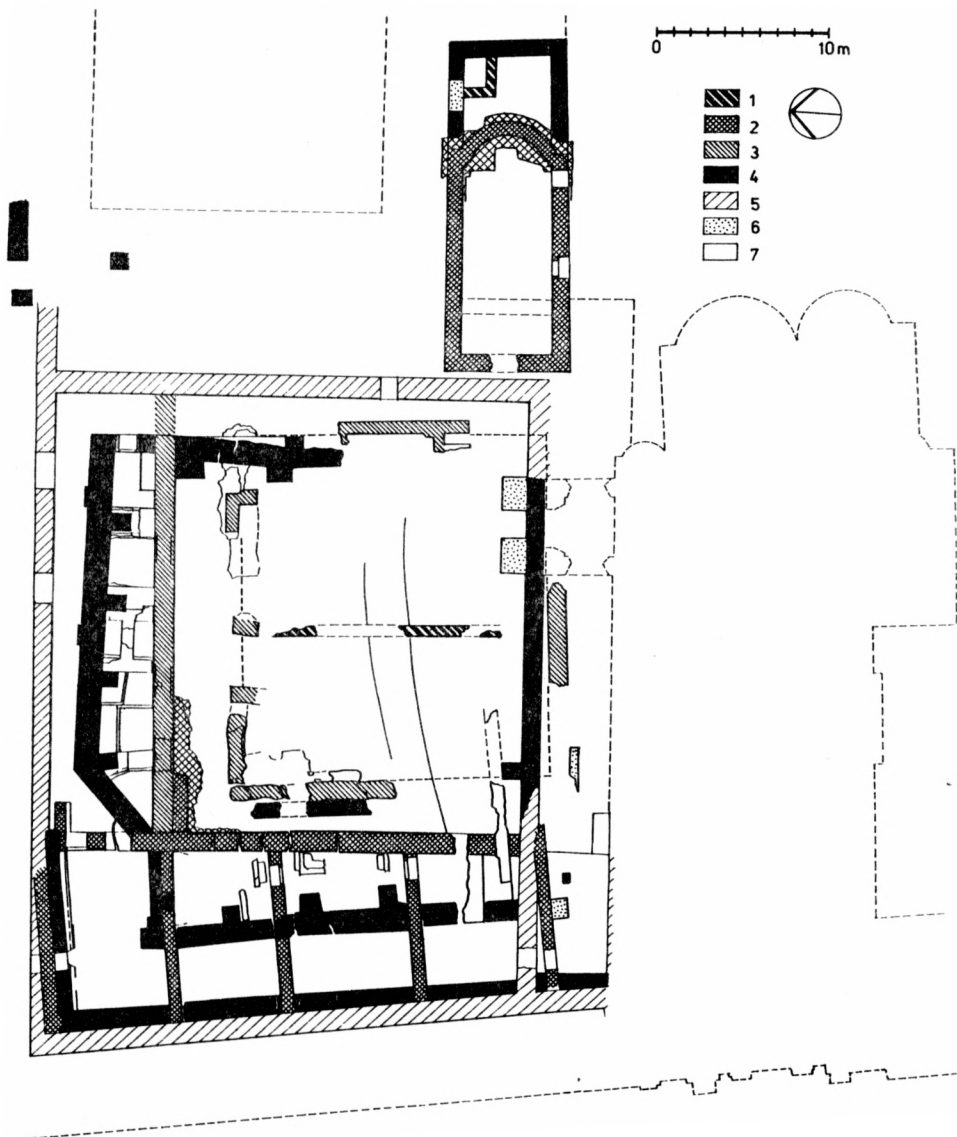
Obr. 2. Pražský hrad, klášter sv. Jiří, Pádorys zdiv klášterních budov, zjištěných archeologickým výzkumem. 1 — předrománské zdivo (?), 2 — románské zdivo — (řidší šraflurou vyznačen předzáklad), 3 — raně gotické zdivo, 4 — vrcholně gotické zdivo, 5 — raně barokní zdivo, 6 — novodobé zdivo, 7 — neurčeno.
