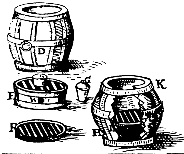
Obr. 13. Pec, v níž se obvykle dělávají méděné průby (Ercker 1974, obr. s. 171, text s. 172: „...pícka z hrncířského materiálu, obložená železy D, nožka, která k ní patří E, železný rošt v ní F, kelímeček s průbou G, větrní otvor, jímž prochází dmychadlo H, celá pec se dnem, jak vyhlíží uvnitř K...“).
