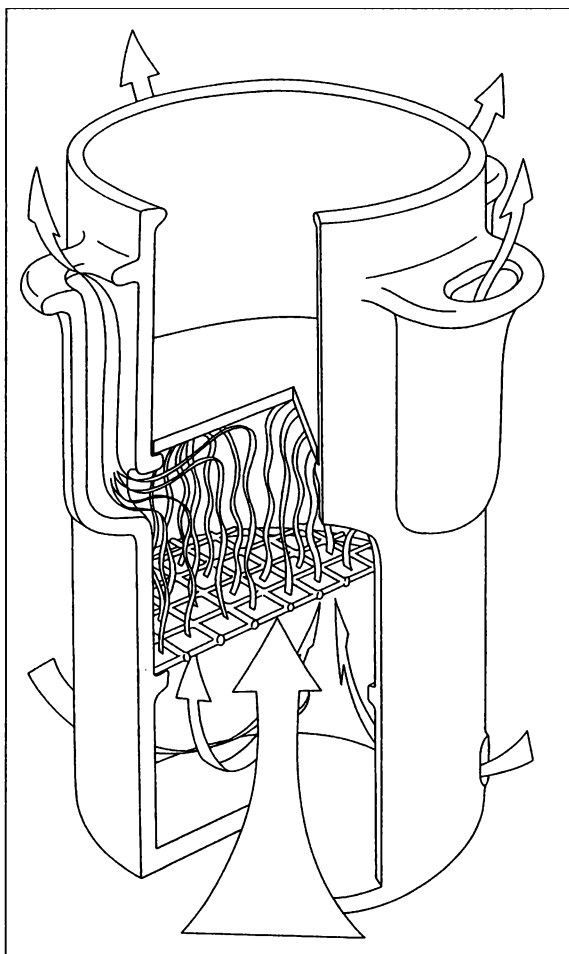
Obr. 3. Č. Krumlov, Radniční čp. 27. Interpretací kresebná rekonstrukce původního vzhledu a funkce jednotlivých částí přenosné keramické pícky. Kresba autor.
