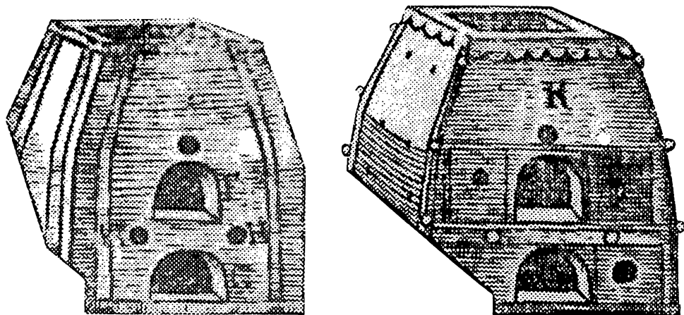
Obr. 5. Prubířské pícky (Ercker 1974, obr. s. 19), vlevo „prubířská pec, zhotovená z hrnčířské hlíny a železnými dlahami sepnutá (op. cit., 20), vpravo „železná prubířská pec, zhotovená z hlazeného plechu“ (op. cit., 20).
