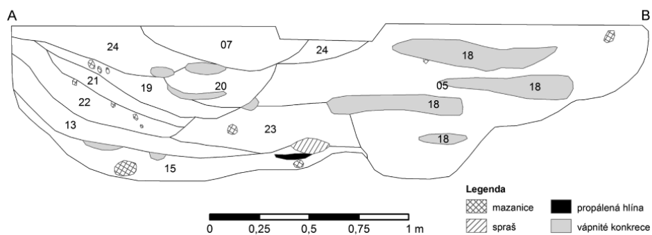
Obr. 2. Těšetice-Kyjovice „Sutny“. Půdorys a profil obj. 738.
