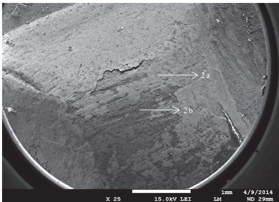
Obr. 5. Mikrosnímek detailu čtvercové kazety zlomku kovového pásu, místo nálezu Brno – Františkánská ulice. Na povrchu je zřetelné poškození postříbřené vrstvy na středu pyramidy. Čísla vyznačují místa měření chemického složení mikrosondou SEM-EDS. Abb. 5. Mikroaufnahme eines Details einer quadratischen Kasette des Metallbandfragmentes, Fundort Brünn – Františkánská-Str. An der Oberfläche ist die Beschädigung der versilberten Schicht auf der Pyramide erkennbar. Die Zahlen kennzeichnen die Messstellen der durch REM-EDX-Analyse ermittelten chemischen Zusammensetzung.
