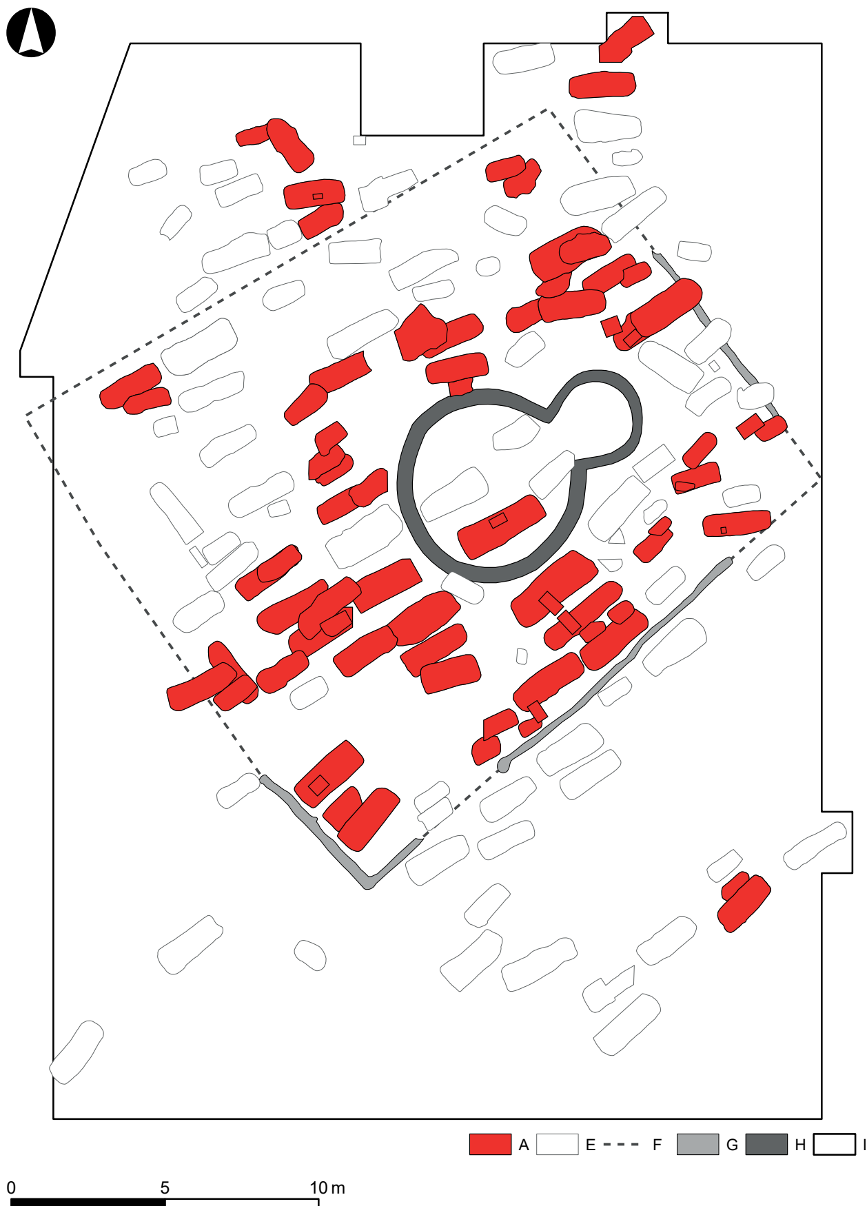
Obr. 94. Břeclav – Pohansko, Severovýchodní předhradí. Plán s vyznačením polohy hrobů ve vzájemné superpozici. Legenda: A – hroby ve vzájemné superpozici, E – ostatní hroby, F – rekonstrukce ohrazení, G – dochované ohrazení, H – základy kostela, I – prozkoumaná plocha.
