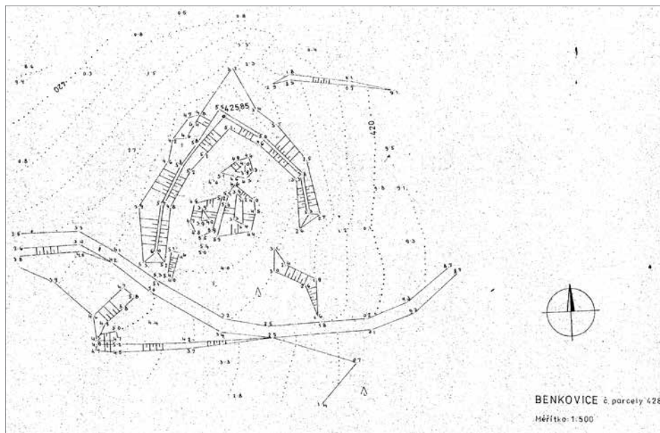
Obr. 3. Opevnění v poloze Před Hanuší v Benkovicích, které tvořilo nejdále severozápadním směrem vysunutě postavení hradeckých sancí. Podle Lissek–Stoklasa 1988. Archiv NPÚ.
