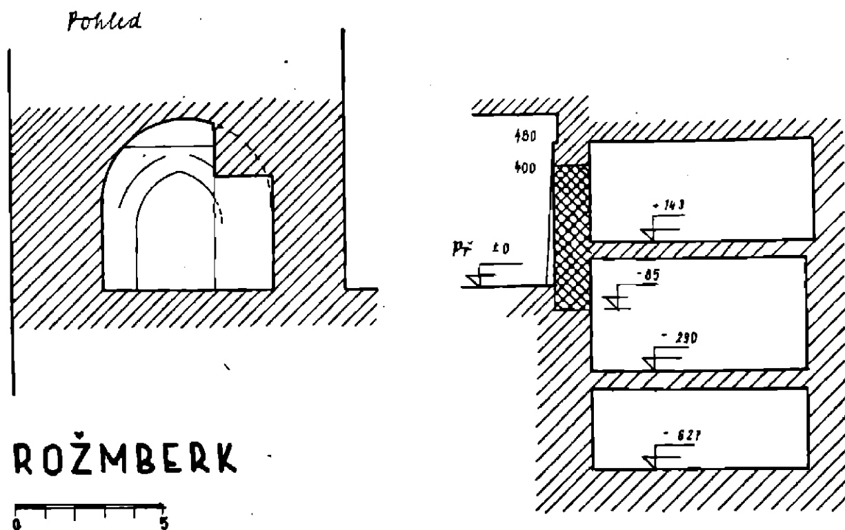
Obr. 2. Rožmberk – dolní hrad. Situace zrušené brány, pohled, řez.
