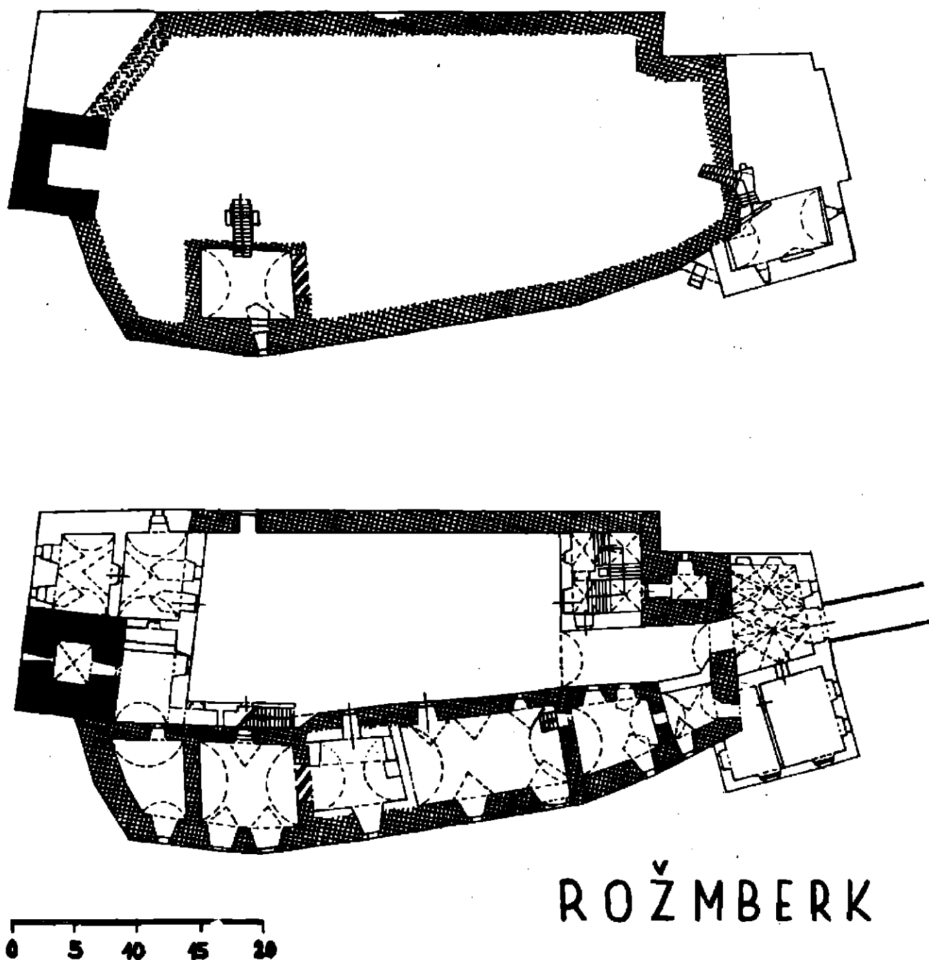
Obr. 1. Rožmberk - dolní hrad. Černě zdivo románské, křížkované gotické sklepy a přízemí.
