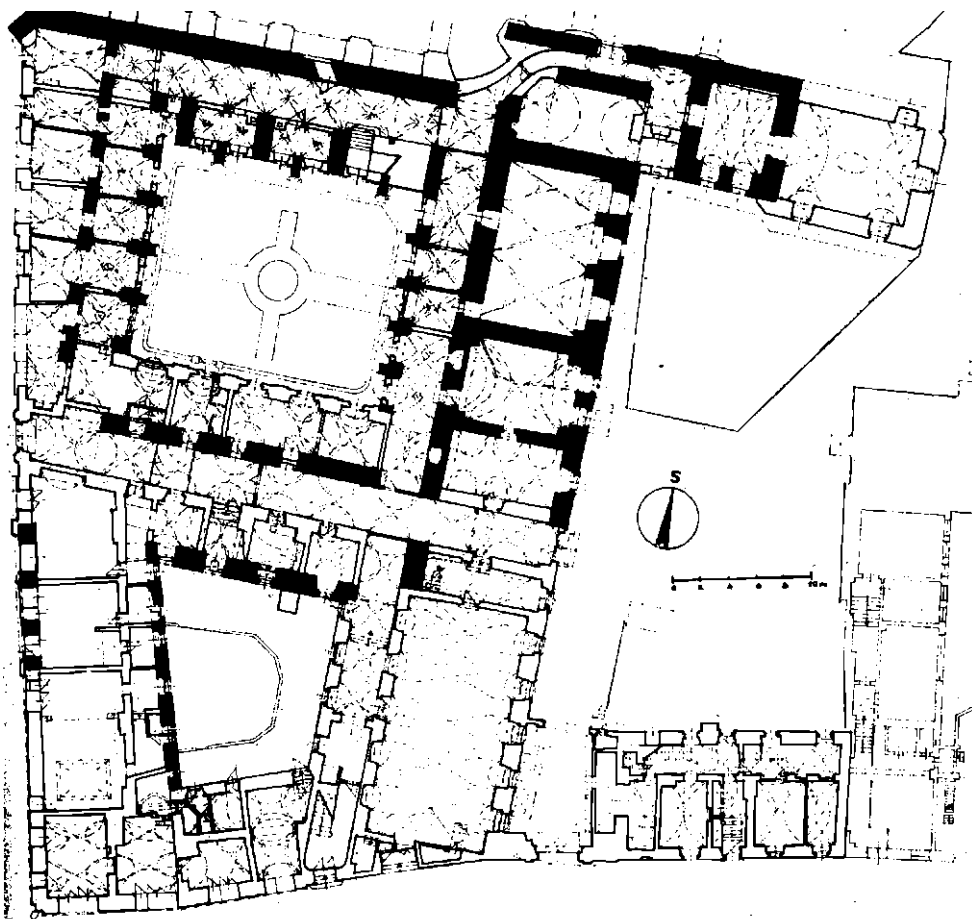
Obr. 1. Minoritský klášter v Brně 1:200. Černé položené zdivo gotické. Nebarevné zdivo barokní a mladší.
