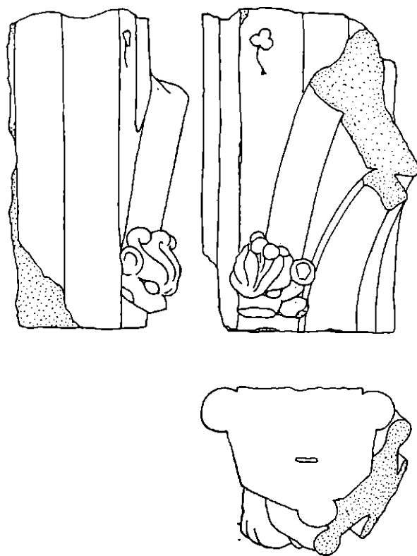
Obr. 1. Lapidarium Pražského hradu, zoomorfní komolka, pískovec, z katedrály sv. Víta (líná vřetenově schodišti). D vlech obrázků jsou tečkovanými plochami označena poškozená místa, grafická měřítká představují délku 10 cm.
