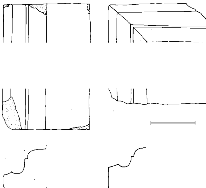
Obr. 7. Soubor goticko renesančních terakotových článků. Ukázky profilovaných soklových desek.
