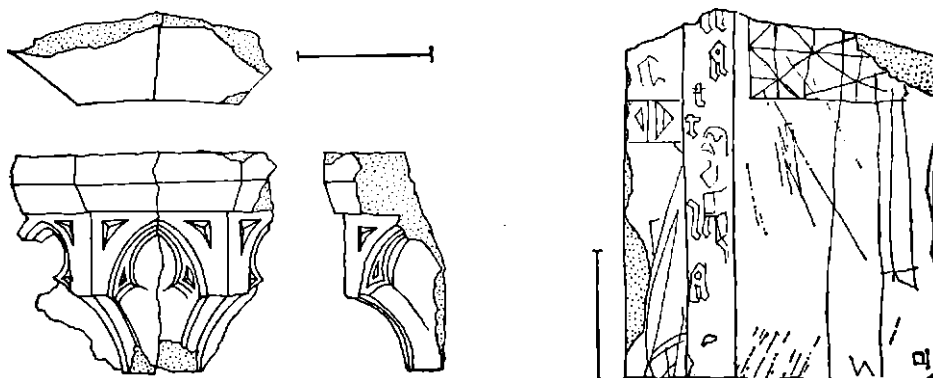
Obr. 2. Kruibová konzola, opuka. Původ neznámý.
