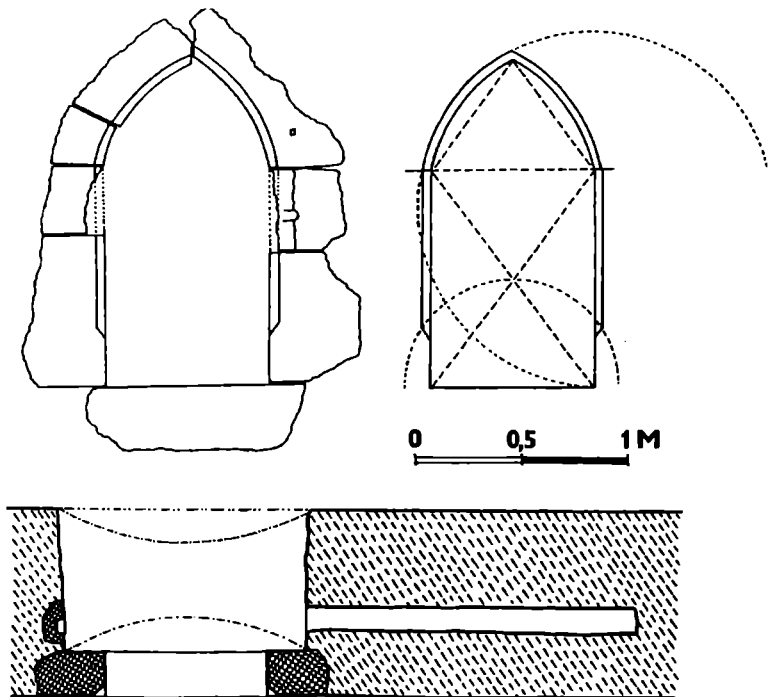
Obr. 5. Bojnice – hrad, ranogotický portál a jeho kompozičná analýza. Kresba M. Bóna.
