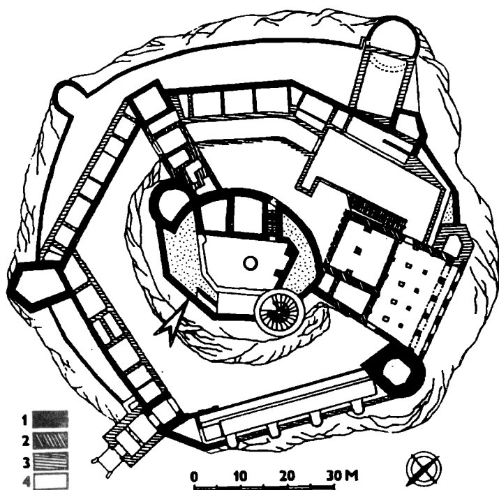
Obr. 2. Bojnice – hrad, situácia hradu so stavebnou etapizáciou podľa D. Menclovej a s označením Archívneho krídla (1– koniec 13. stor.–zač. 16. stor.; 2 – 2. pol. 16. stor.; 3 – pol. 17. stor.; 4 – 19. stor.). Kresba M. Bóna.
