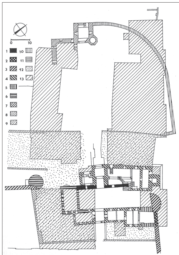
Obr. 11. Kolín. Rekonstrukce situace hradu (bez vodní věže – soukres půdorysy současného stavu a historických plánů). 1 – dochované zdivo městské hrady z 13. století, 2 – zdivo téže hrady dochované v úrovni suterénu, 3 – zdivo městského opevnění doložené historickými plány, 4 – dochované zdivo hradu z konce 30. let 15. století (u jihovýchodního křídla s možným využitím zdiva staršího kláštera), 5 – zdivo hradu jádra dochované v úrovni suterénu, 6 – zdivo jádra hradu doložené historickými plány, 7 – historickými plány doložené snad středověké zdivo jádra hradu, 8 – historickými plány doložené eskarpová (tj. linie parkánové hrady městského opevnění) a kontreskarpová zed příkopů, 9 – dochované pozdně gotické zdivo předhradí, 10 – historickými plány doložené opevnění předhradí, 11 – patrně pozdně gotické zdivo v jádře, 12 – historickými plány doložená plocha příkopů, 13 – současná zástavba. Kresba autor.
