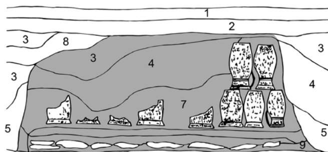
Obr. 14. Hrnčířská pec z Horšovského Týna. 1 – půdorys pece na hraně výkopu, 2 – řez stěnami pece včetně umístění keramických nádob; popis uloženin: 1 – chodník z dlaždic, 2 – vyrovnávací štěrkopísková navážka, 3 – destrukční vrstva pece, 4 – mazanice se zlomky nádob, 5 – žlutka, uhlíky, zlomky keramiky, 6 – jílovité podloží, 7 – keramika uložená v mazanici, 8 – hlinito-písčítá vrstva s obsahem zlomkové keramiky, 9 – přepálená žlutka s kameny základu pece. Podle Frýda 1992, Tab. IV a V, upravil L. Čapek.
