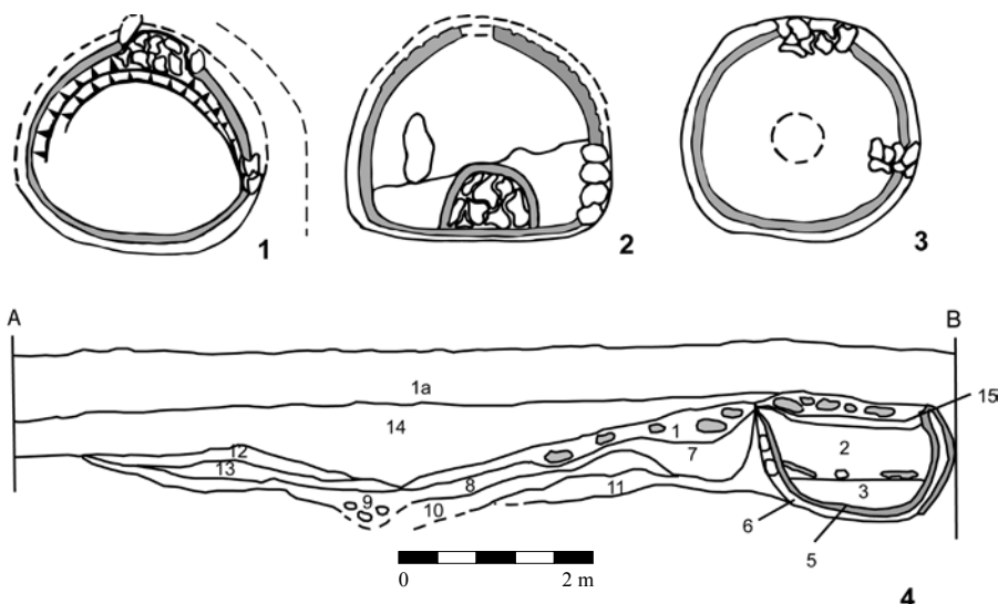
Obr. 10. Hrnčířská pec z Tábora – Sídliště nad Lužnicí. 1 – půdorys dna, 2 – boční pohled, 3 – pohled ze shora, 4 – řez peci včetně předpecní jámy; popis uloženin: 1 – hnědočerná hlinitá s kameny – navážka, 1a – hnědá hlinitá s cihlovou drtí a kameny – navážka, 2 – hnědá hlinito-písčítá, 3 – černá propálená s mazanicí a cihlovinou, 5 – šedočerná mazanice z vnitřní vyzdívkou klenby pece, 6 – cihlově červený vnější plášť pece, 7 – šedočerná hlinitá v předpecní jámě, 8 – černá uhlíková, 9 – zahloubení do vrstvy 8, složením analogická, 10 – žlutá hlinitojílovitá s uhlíky, 11 – hnědá hlinitá, 12 – šedá jílovitá s kameny, 13 – šedo hnědá jílovitohlinitá, 14 – hnědá hlinitá s cihlovinou, 15 – černošedá hlinitá. Podle Krajc 1982, obr. 2, upravil L. Čapek.
