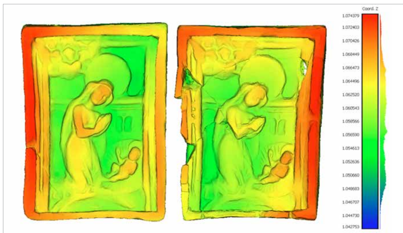
Obr. 17. Vizualizace výškové mapy modelu a rozdílné deformace čelní vyhrávací stěny originálu.
