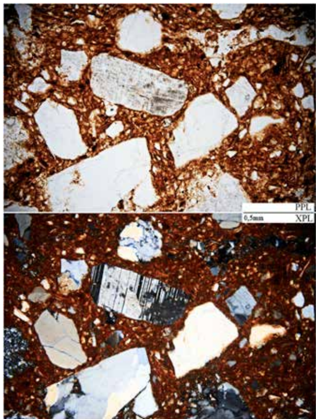
Obr. 4. Cvilín – hrad. 1 – Kachel se sokolníkem a psy (L3, foto M. Tymonová, kresba M. Schindlerová); 2 – úlomek plagioklasu v mikrostruktuře keramického střepu, PPL, XPL.
