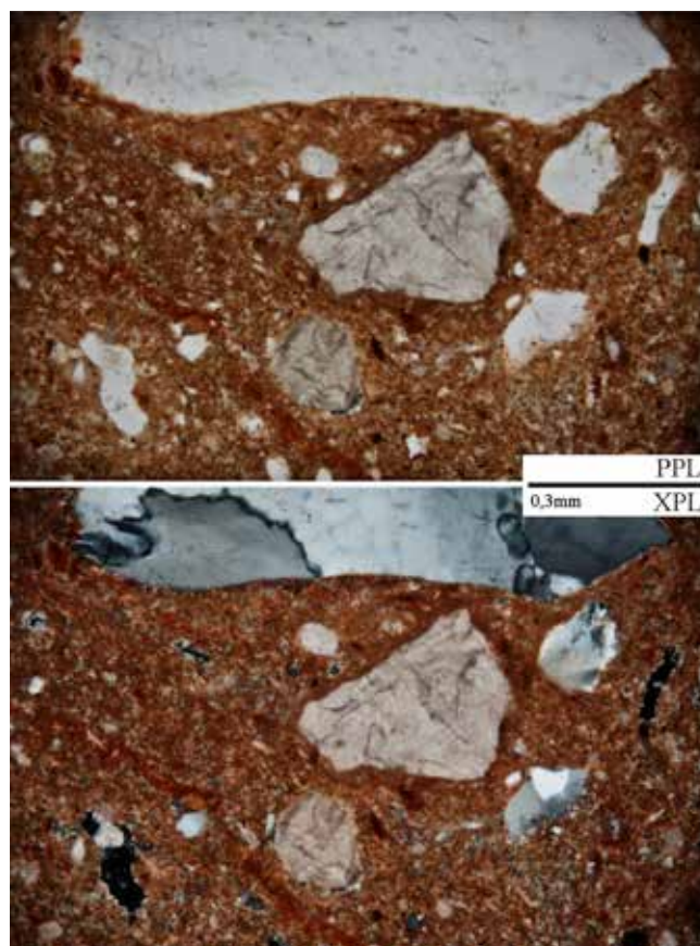
Obr. 5. Štamberk (Šternberk), hrad. 1 – Torzo ženské postavy s rouškou; 2 – úlomky mramorů v mikrostruktuře keramického střepu, PPL, XPL.
