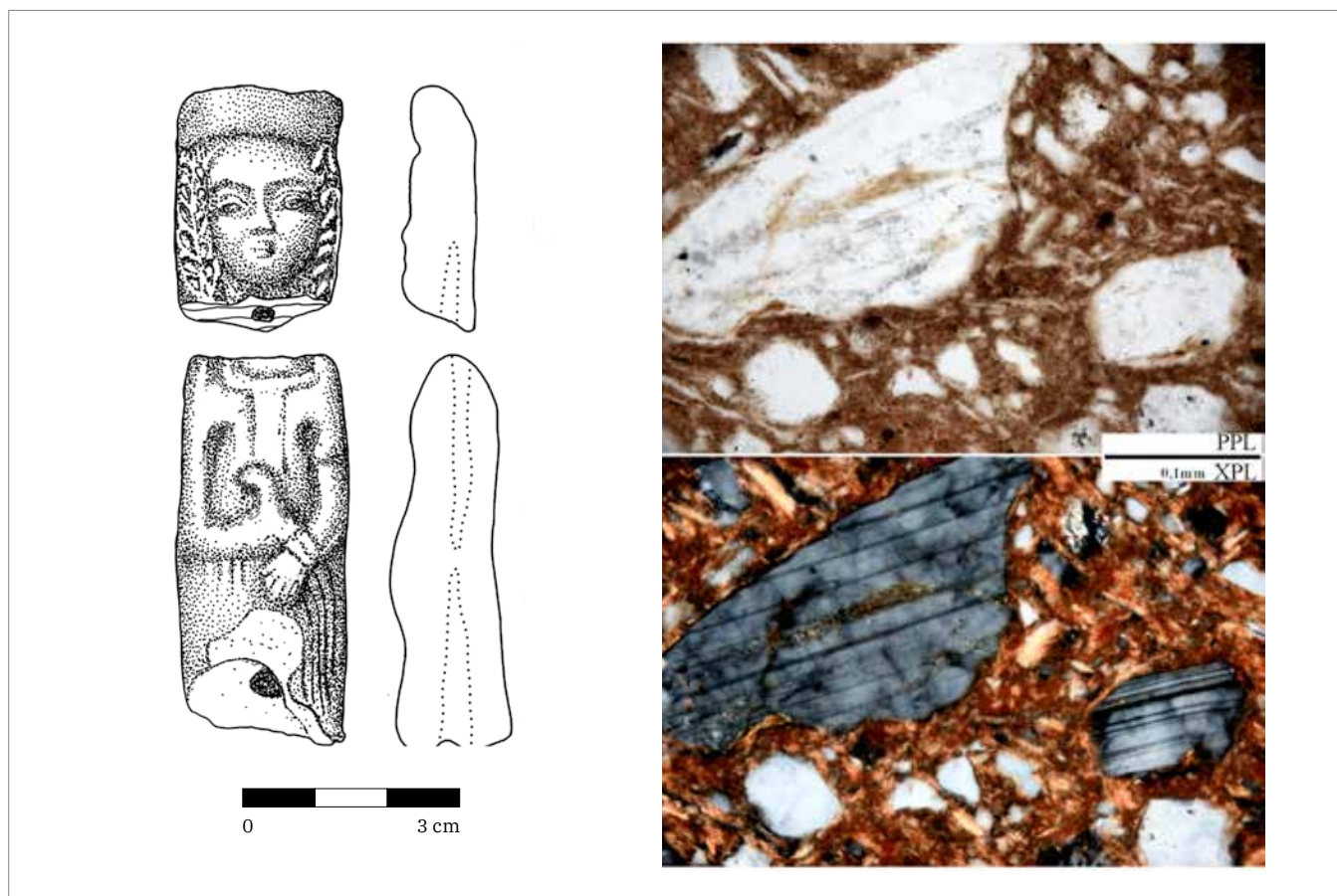
Obr. 28. Bystřec, k. ú. Jedovnice. 1 – Ženská postava (světice?) s neurčitelným předmětem v rukou; 2 – úlomek plagioklasu v mikrostruktuře keramického střepu, PPL, XPL.
