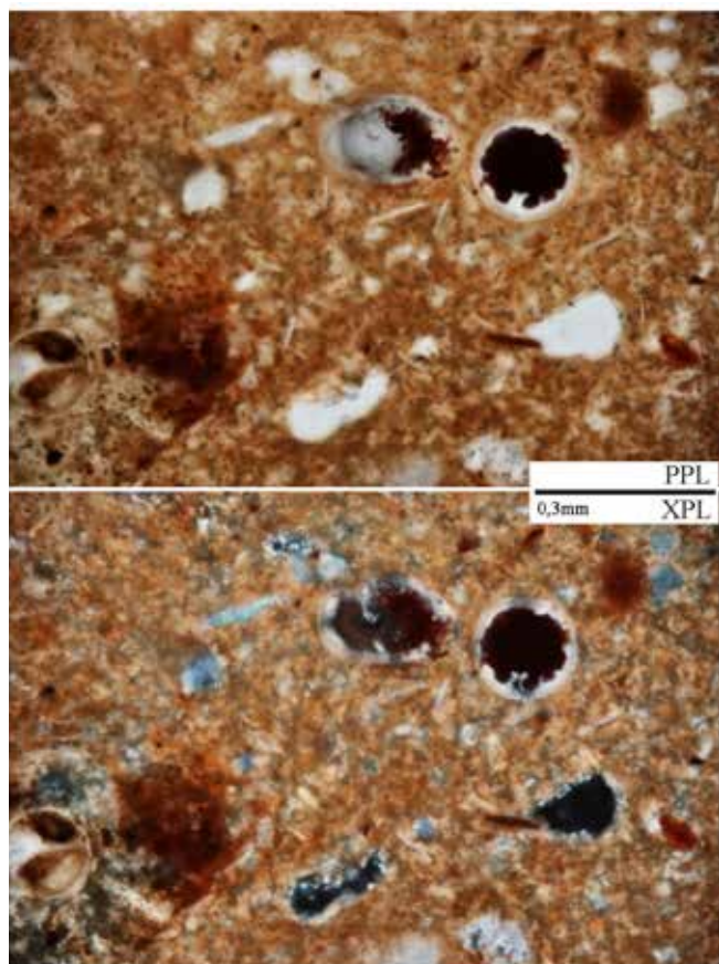
Obr. 1. 1 Mstěnice, dvůr usedlosti 16. 1 – Hlavička ženské plastiky v kruseleru se čtyřnásobným vinutím; 2 – mikrofosilie v mikrostruktuře keramického střepu, PPL, XPL.
