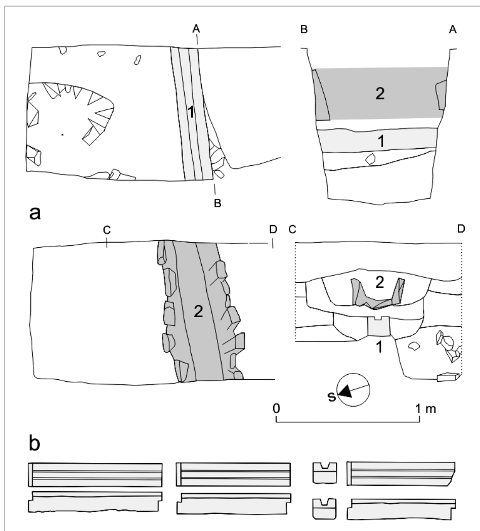
Obr. 10. Kresbová dokumentácia superpozície kamenného barokového vodovodu a kamenno-maltového žľabu z 20. storočia (a) a odkrytých kamenných žlábkov (b). Digitalizácia M. Samuel.
