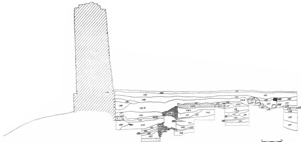
Obr. 3. Stará Boleslav. Sonda W, východní řez. Kontexty 4153, 4148, 4147 — původní půdní horizont; 4904 — čelní plenta valového opevnění; 4149 — zbytek tělesa valu (?); 4146, 4150, 4151 — planýrky; předcházející výstavbě zdi 4901A; 4131, 4114 — stavební vrstva ke zdi 4901A; 4901B — mladší rozšíření. Kreslil J. Frolík.
