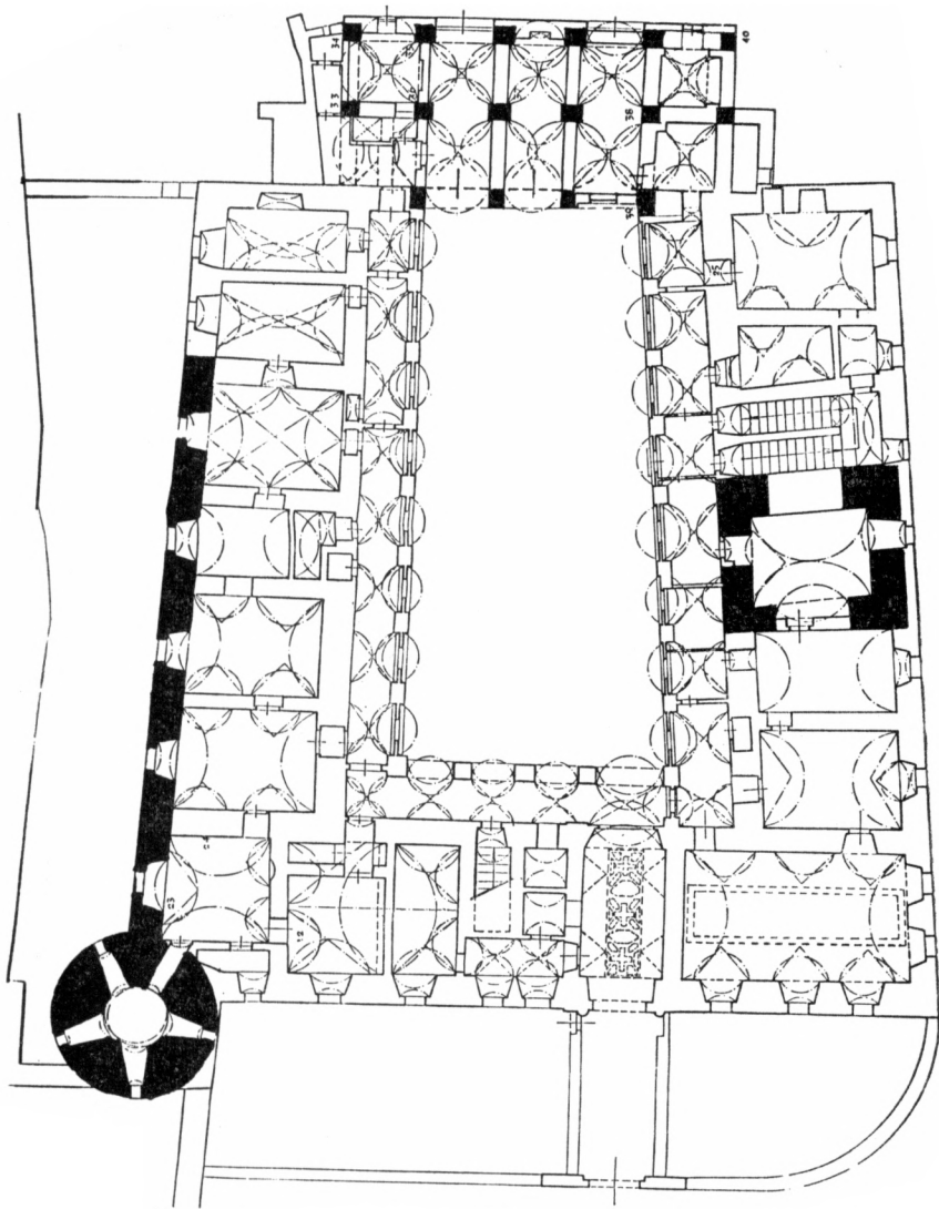
Obr. 2. Půdorys přízemí zámku v Hranicích s vyznačením starší gotické brány, věže a pravděpodobného zbytku perštejnského hradu, renesančního logglového severního křídla.
