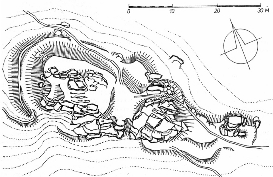
Obr. 7. Hrad Skalný (Hostýnské vrchy) — celkový půdorys.
