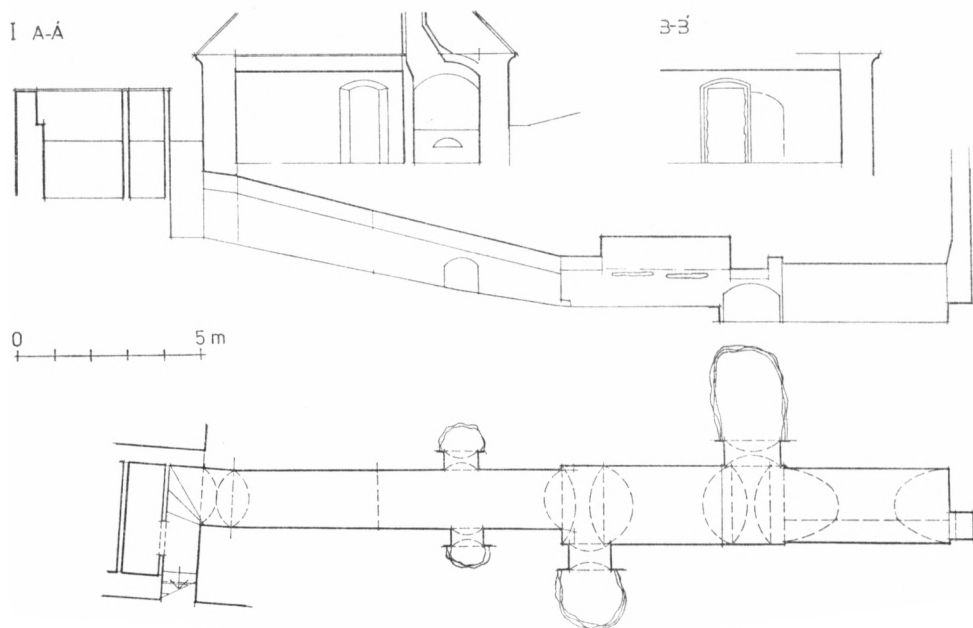
Obr. 16. Vrhavčice, objekty v prostoru bývalé věže, řez a půdorys sklepů. Stav roku 1984 (kresba J. Anderle).
