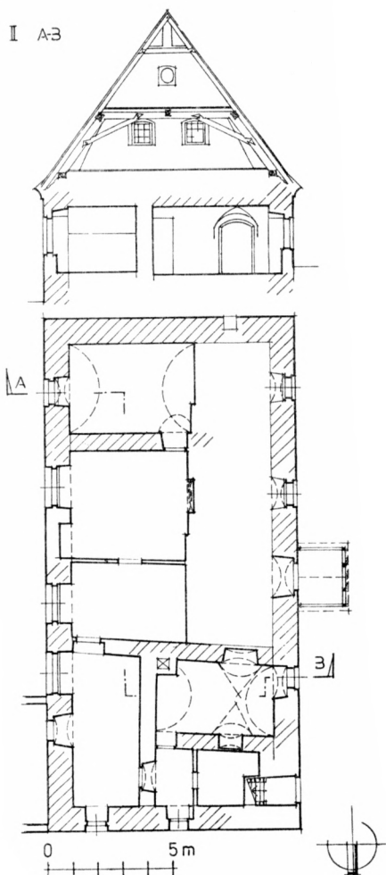
Obr. 12. Vrhavěč, pozůstatek mladší tvrze. Šrafované vyznačeno zdívo pravděpodobně renesanční, stav roku 1984 (kresba J. Anderle).
