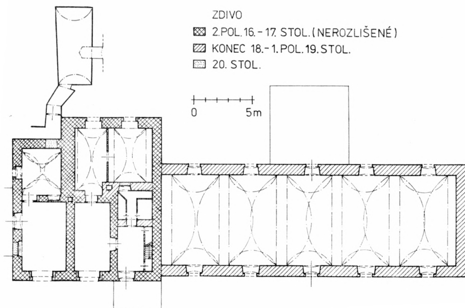
Obr. 7. Kouskova Lhotka, obytné stavení dvora. Zaměření M. Rykl 1986 (obrázky 1—5 a 7 kresba M. Rykl).
