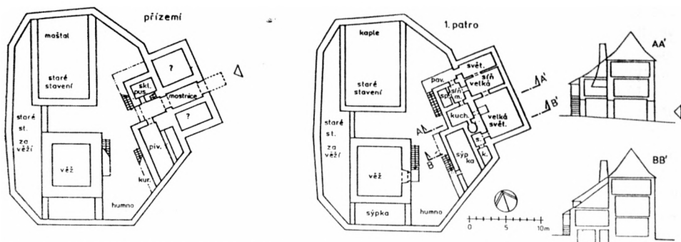
Obr. 4. Kouskova Lhotka, stav tvrze v polovině 17. století. Nejpravděpodobnější varianta situace podle popisu z roku 1635.
