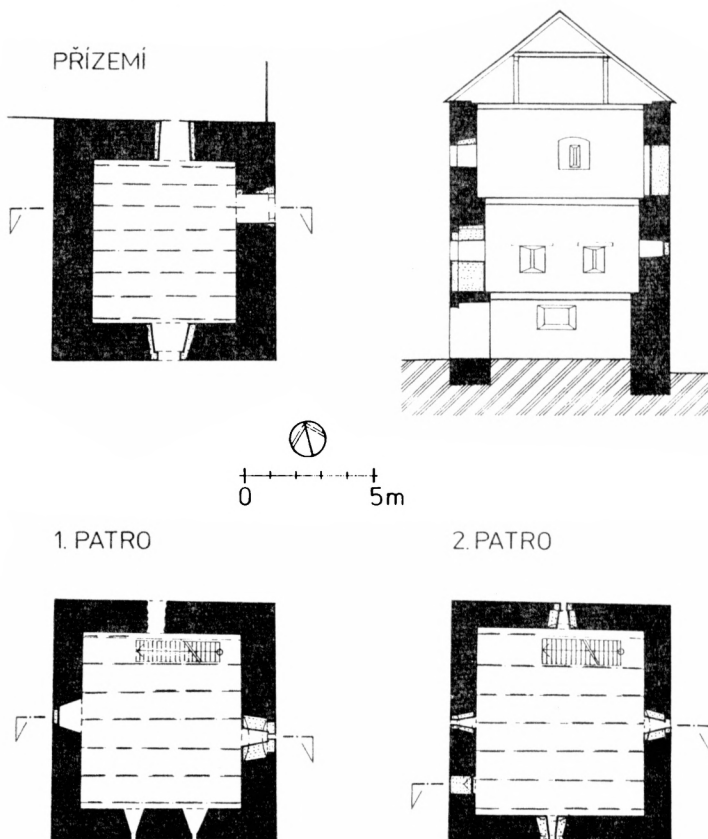
Obr. 5. Kouskova Lhotka, věž tvrze (zaměření M. Rykl a J. Úlovec 1986 až 1992).
