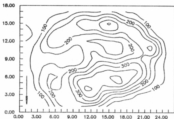
Obr. 7. Radola. Mapa izoohm.
