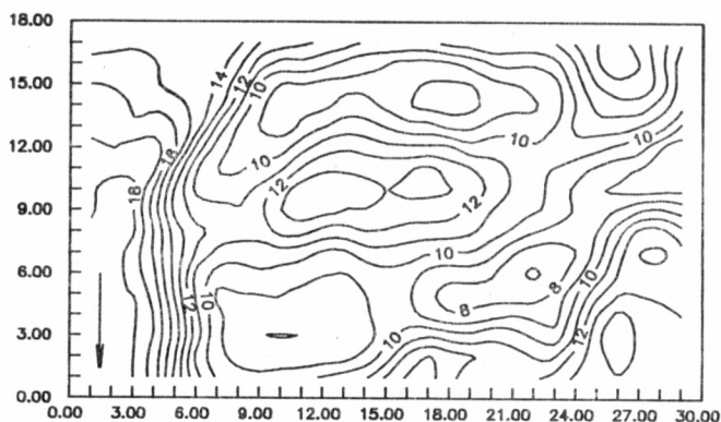
Obr. 8. Radola. Mapa izomliemens.
