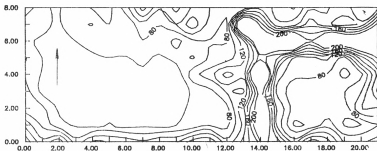
Obr. 5. Lipovník. Mapa izoohm.
