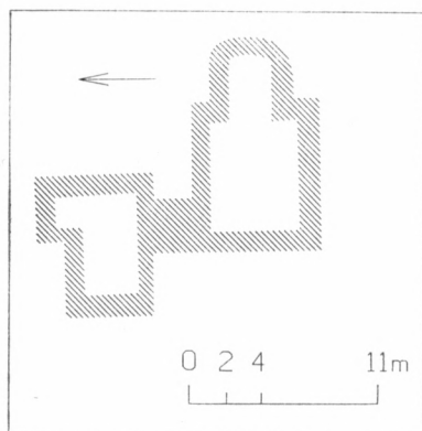
Obr. 15. Veľký Kamenec. Zidealizovaný pôdorys základov múrív.
