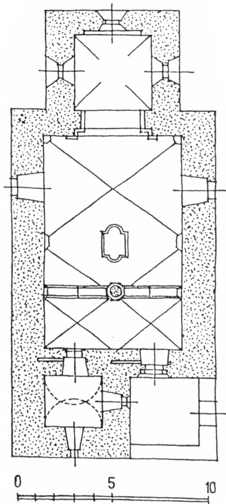
Obr. 1. Kostel Věch svatých v Řesanících, okres Plzeň-jih, půdorys podle E. Šamánkové, doplněno.
