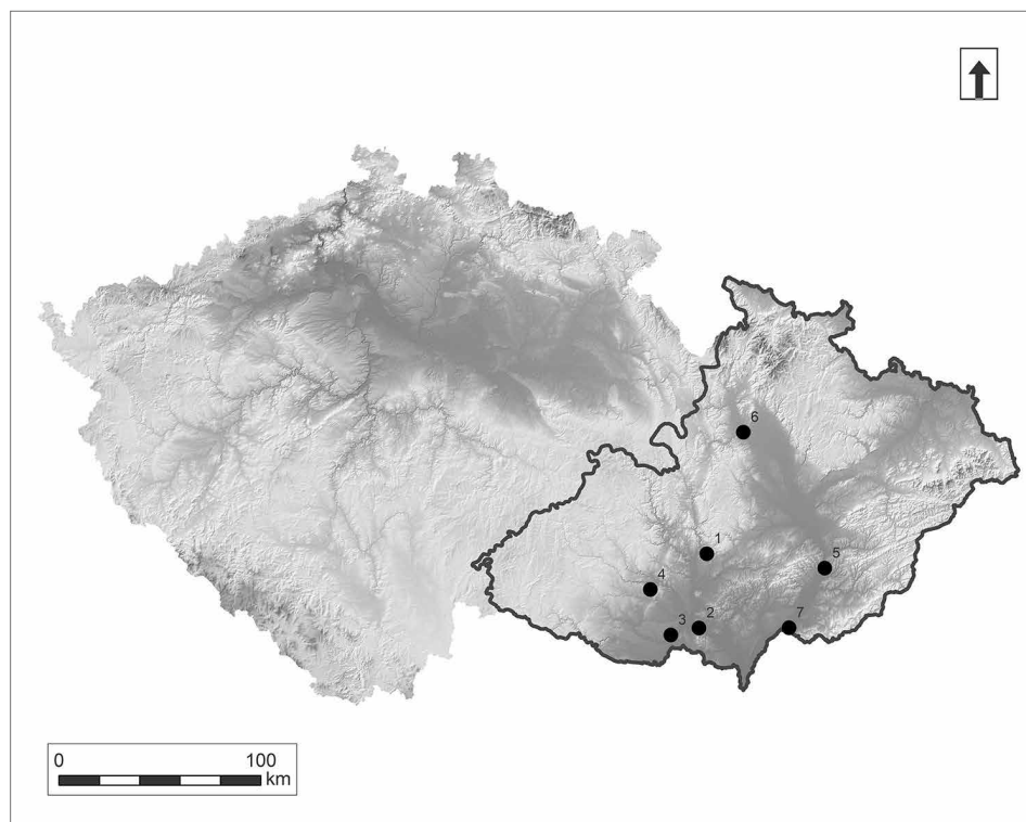
Obr. 1. Geofyzikálně zkoumaná mladohradištní centra na Moravě. 1 – Brno – Staré Zámky; 2 – Dolní Věstonice – Vysoká zahrada; 3 – Drnholec; 4 – Rokytná; 5 – Spytihněv; 6 – Stavenice; 7 – Sudoměřice.
