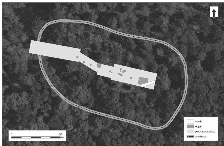
Obr. 7. Drnholec. Archeologická interpretace magnetické prospekce.
