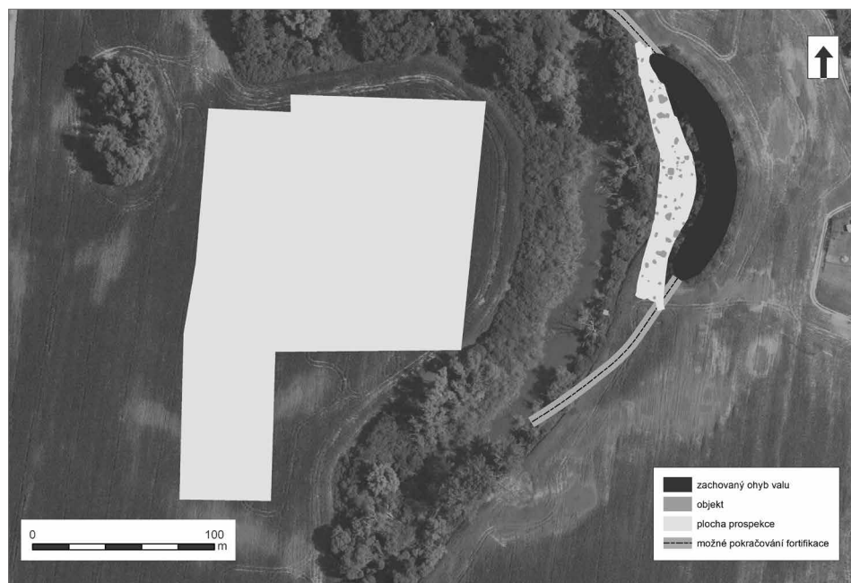
Obr. 12. Spytihněv. Archeologická interpretace magnetické prospekce.
