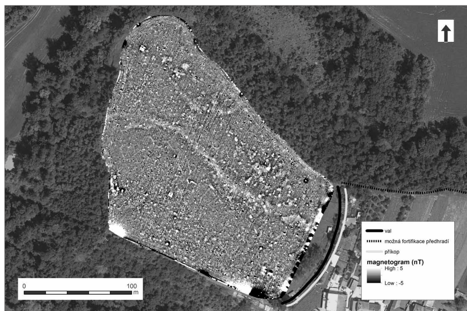
Obr. 9. Rokytňá. Magnetogram prozkoumané plochy akropole hradiska.
